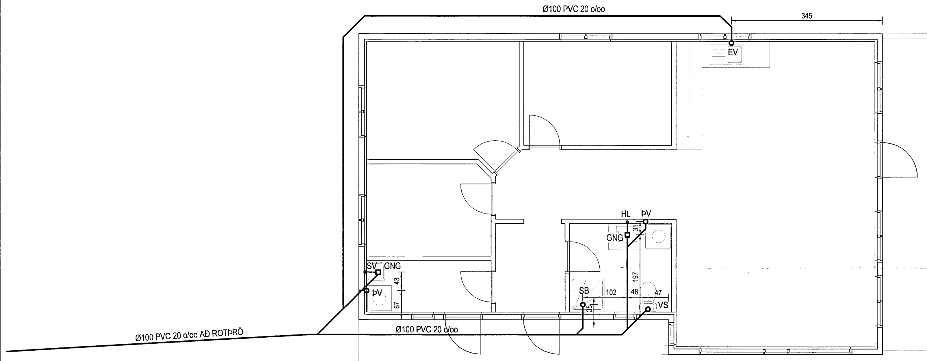
FRÁRENNISLAGNIR GRUNNMYND MKV. 1:50
