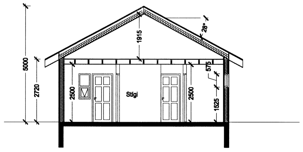
Skurðmynd A-A Mkv. 1:100
