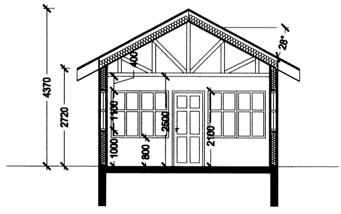
Skurðmynd B-B Mkv. 1:100
