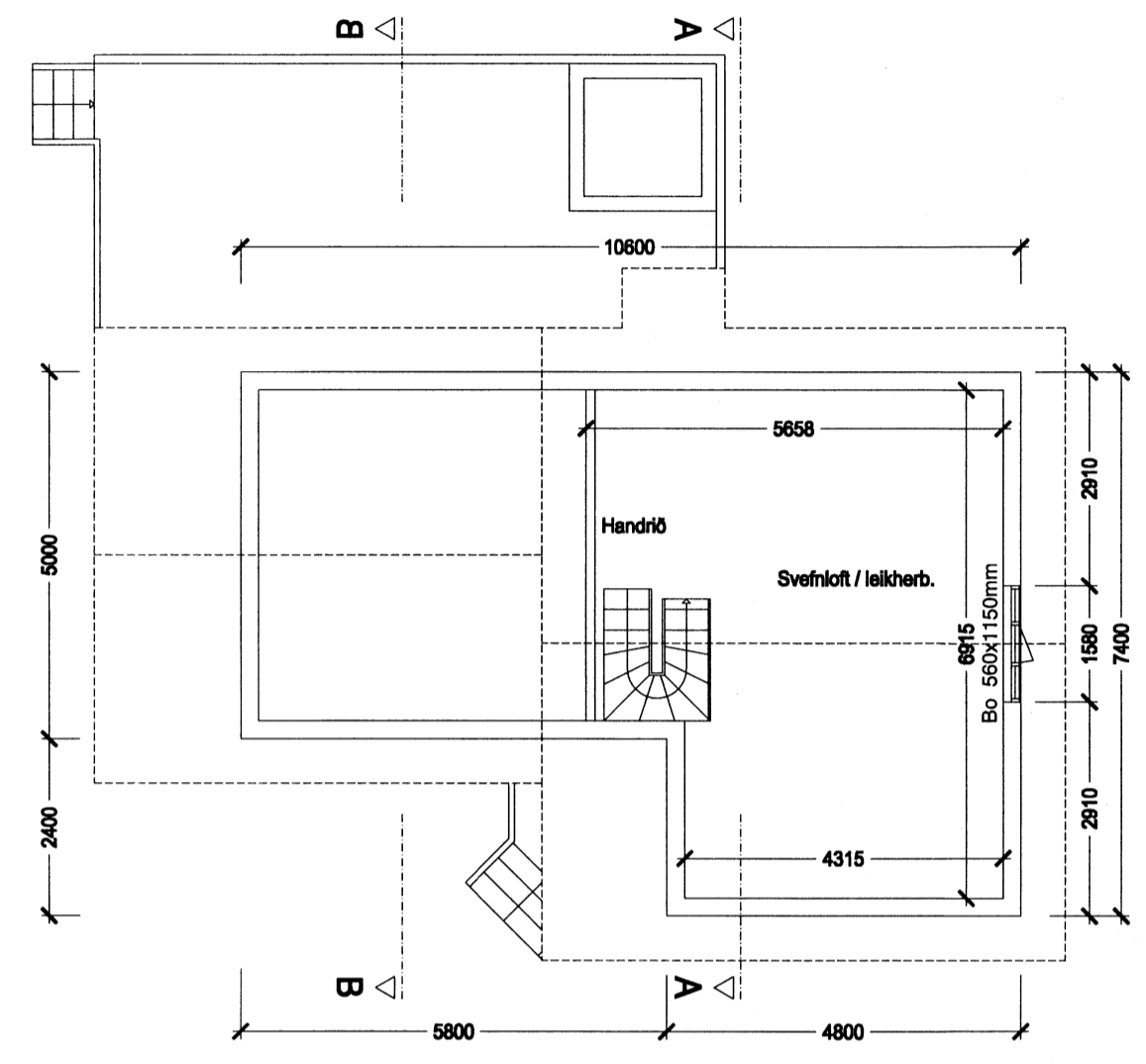
Grunnmynd 2.hæð Mkv. 1:100
