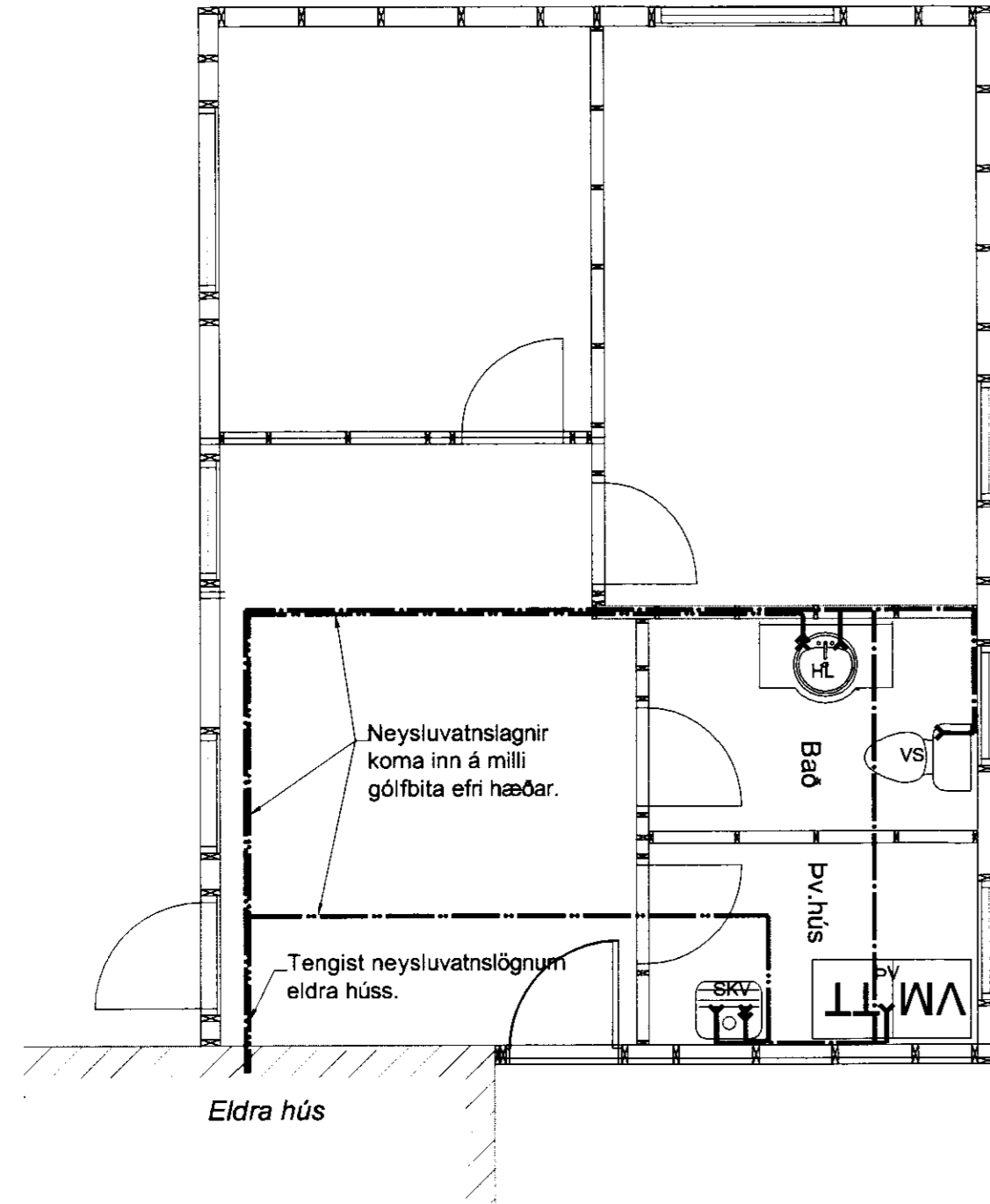
Grundmynd neysluvatnslagna
