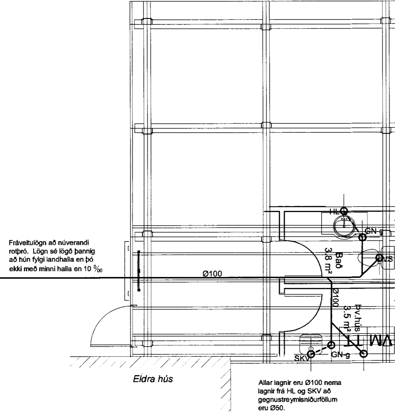
Grundmynd fráveitulagna
