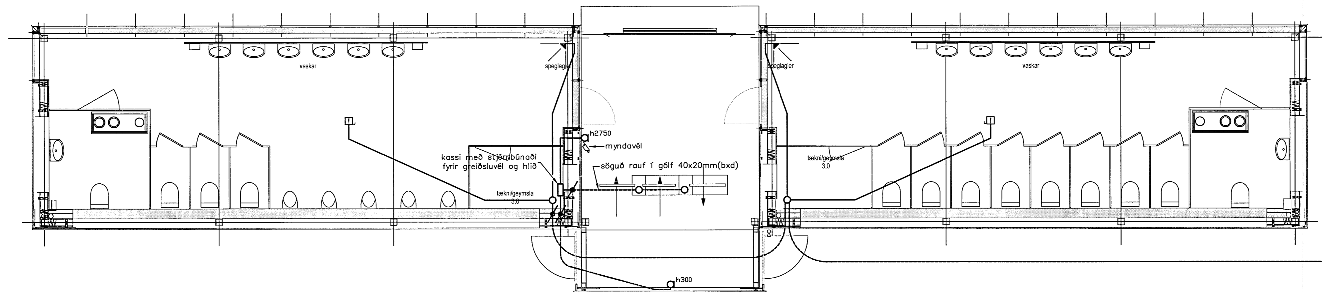
1 GRUNNMYND HÚS 1 - kvennasnyrtingar - mkv: 1:50
