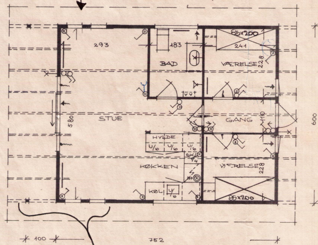
SPEC. ELEMENTTEGNING
