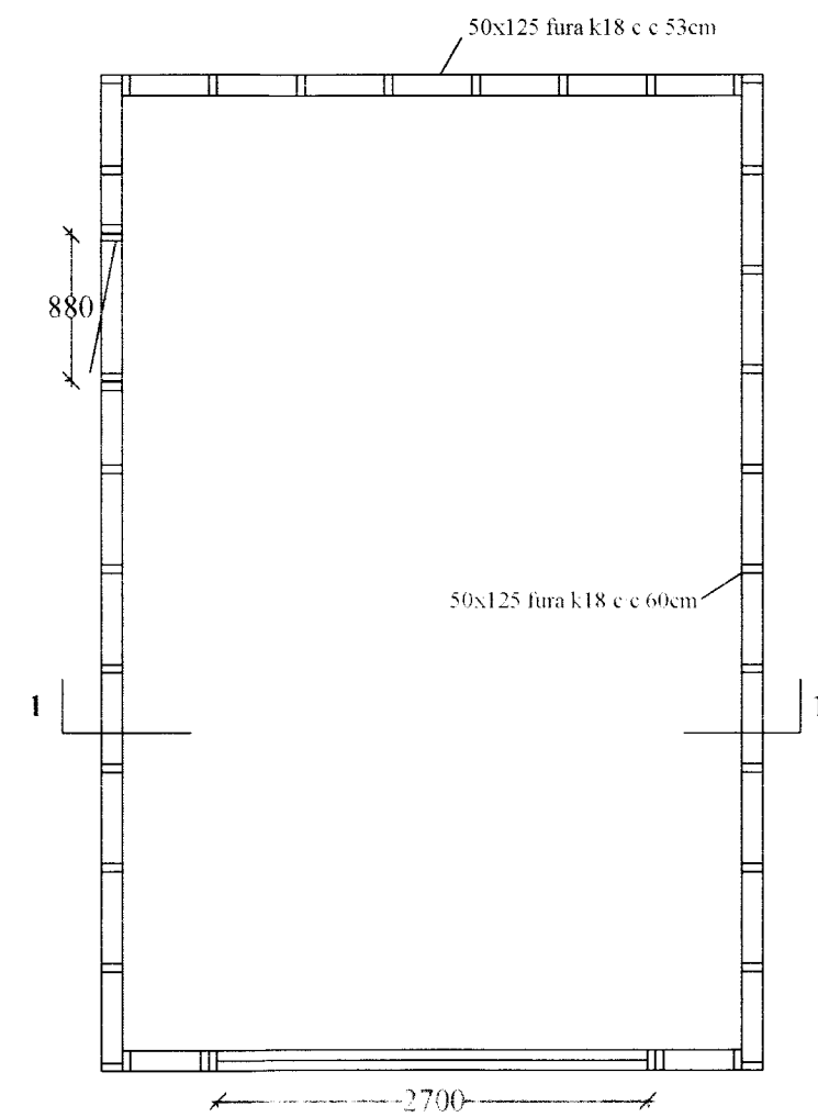
Veggir M 1:50
