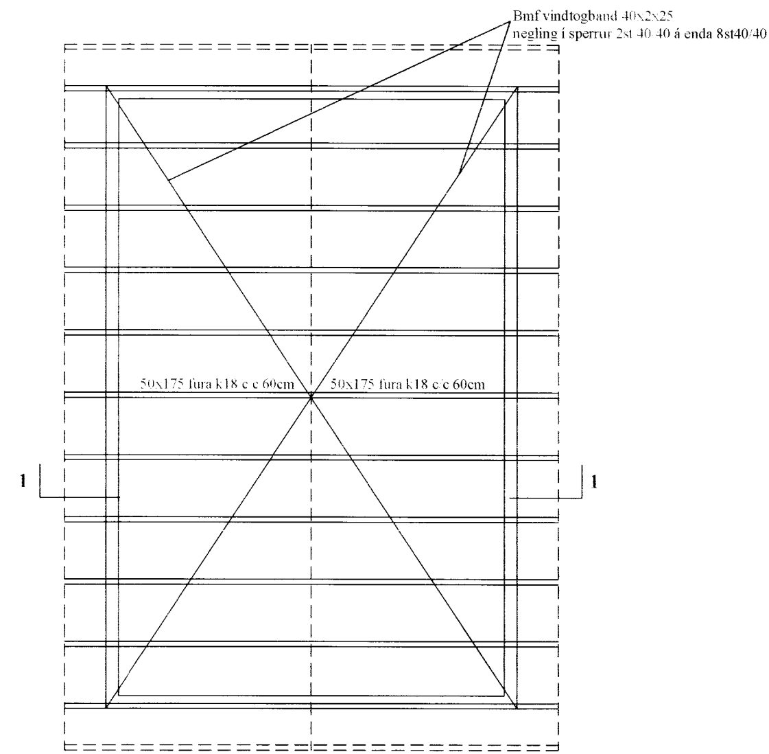
Þak M 1:50
