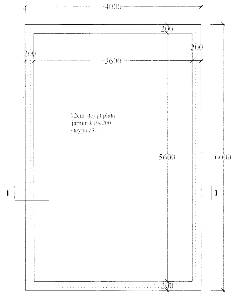
Undirstöður M 1:50
