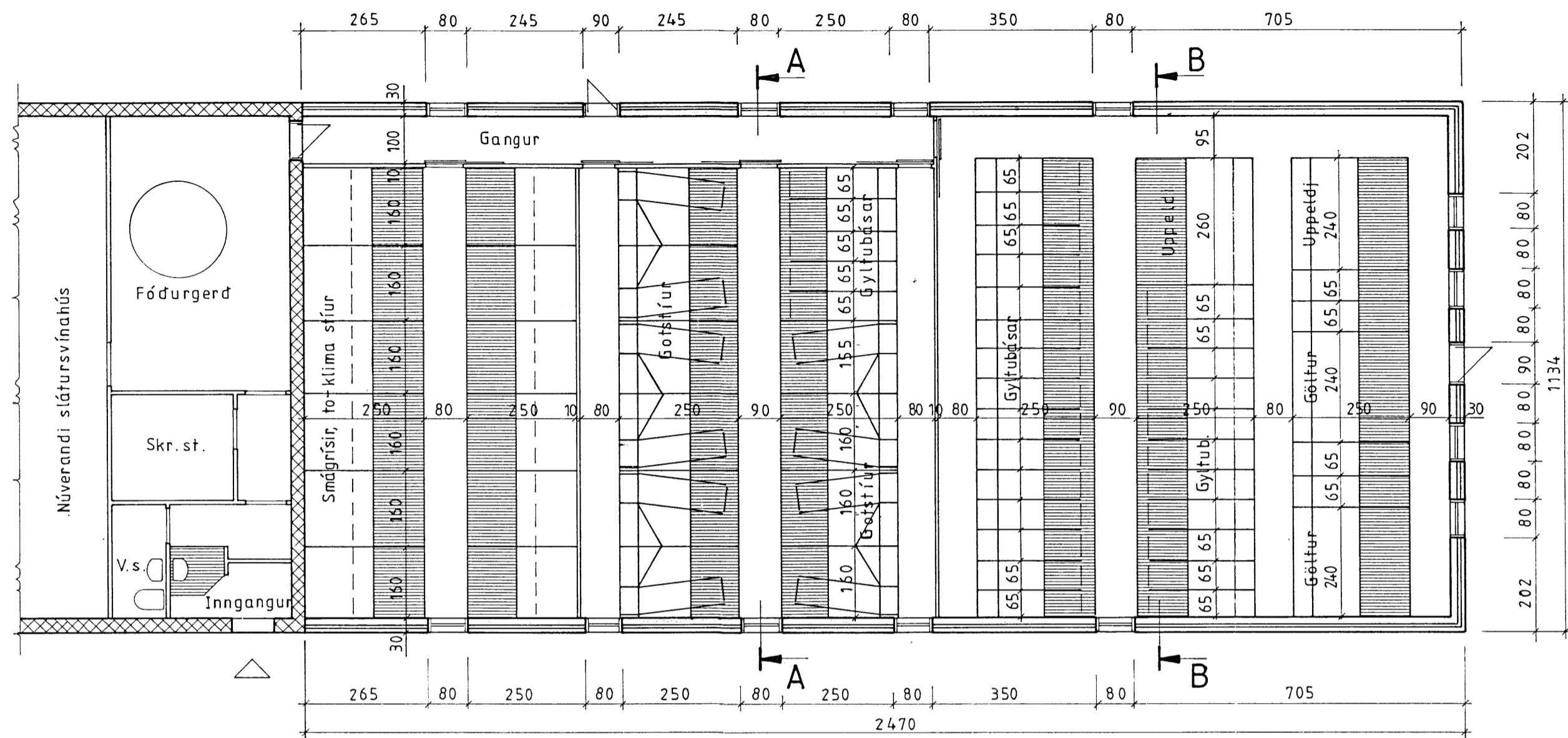
Grunnmynd.
