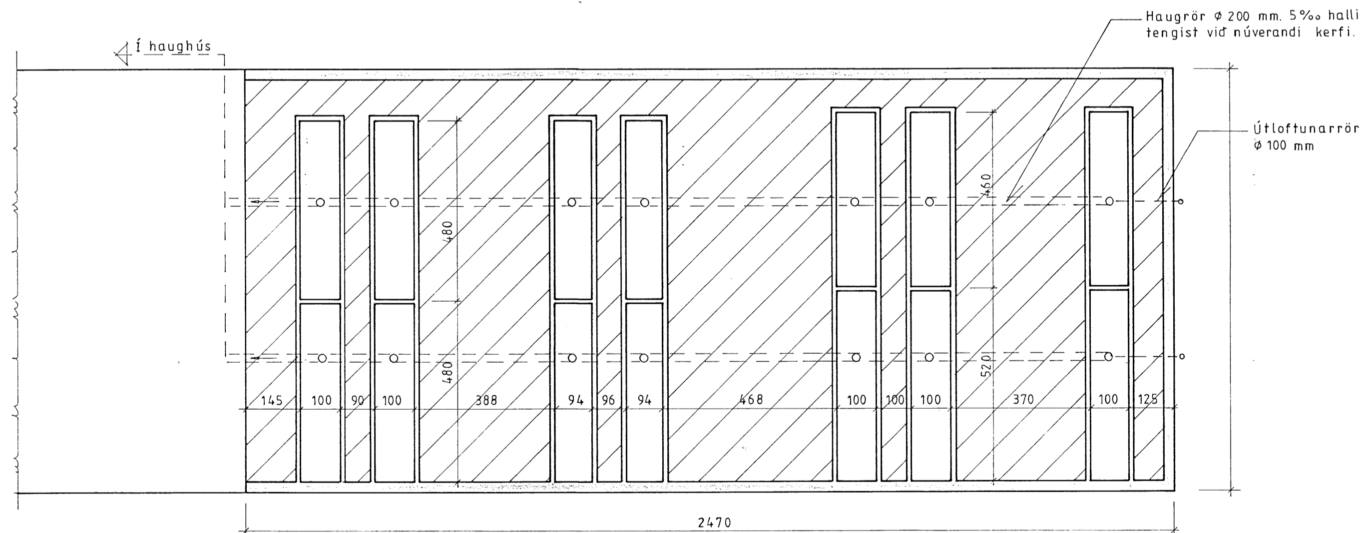
Sökkjar/Flórar.
