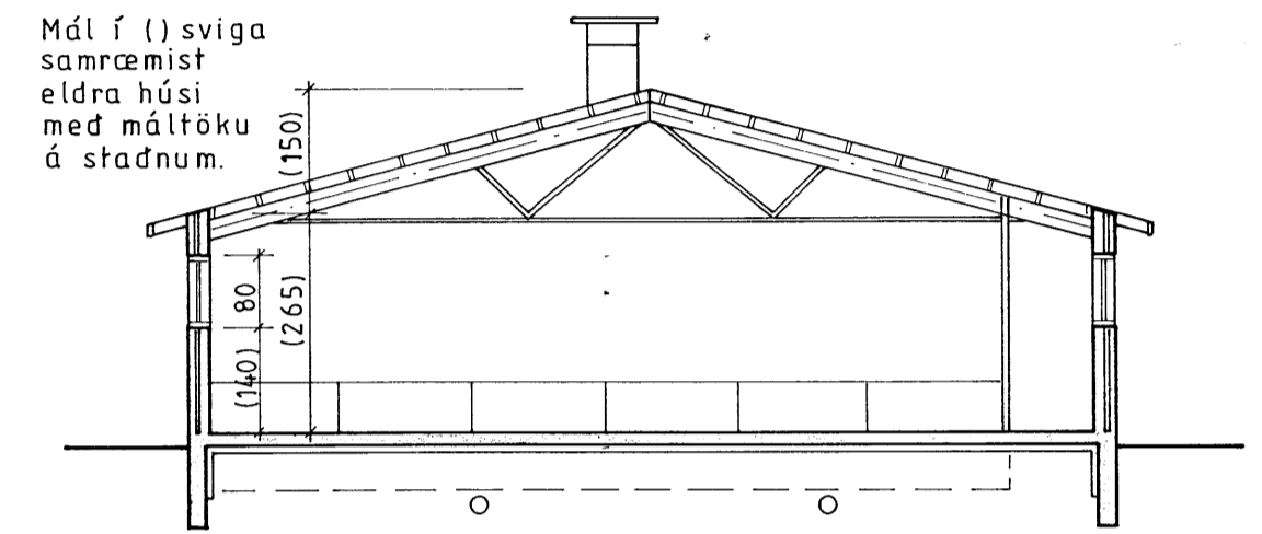
Snid A-A
