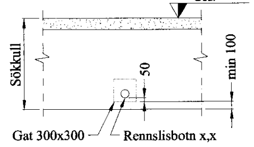
Skýringamynd af sökkulgötum GK:
