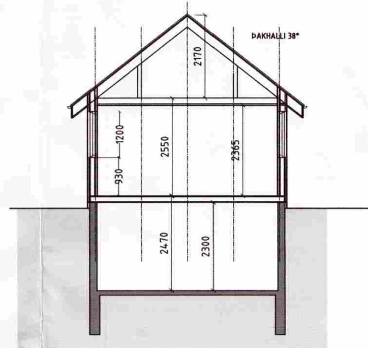
SNEIÐMYND A-A
