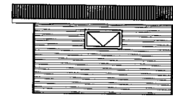
Austur 1:100 (garðskúr)
