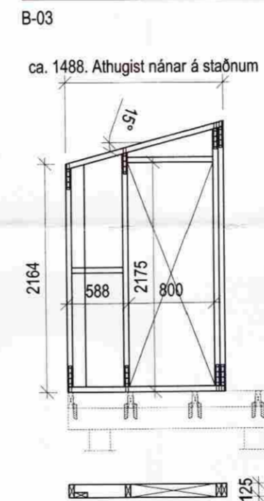
Grind 6 Mkv. 1:50
