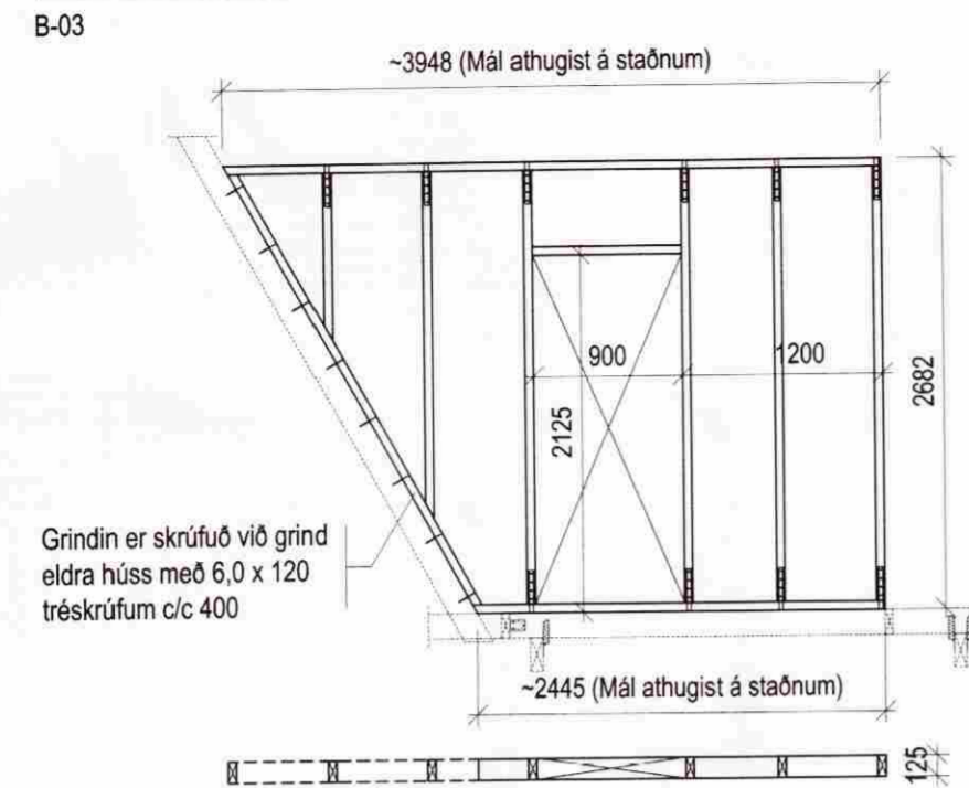
Grind 1 Mkv. 1:50
