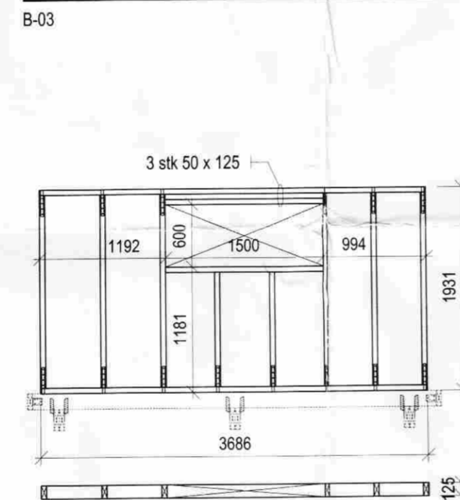
Grind 5 Mkv. 1:50
