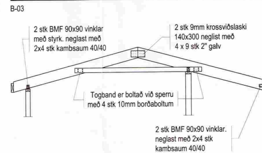
Snið Þ1 Mkv. 1:50
