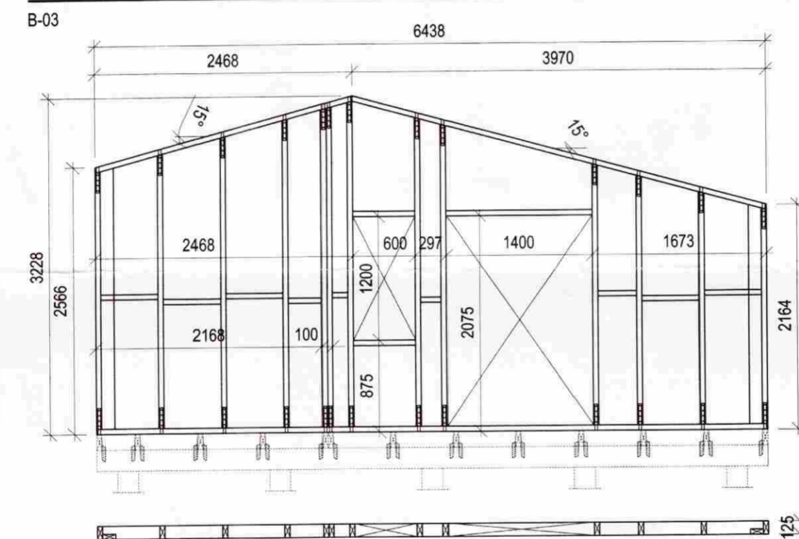
Grind 4 Mkv. 1:50
