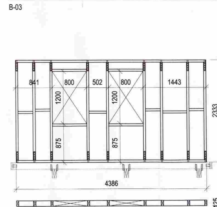
Grind 3 Mkv. 1:50
