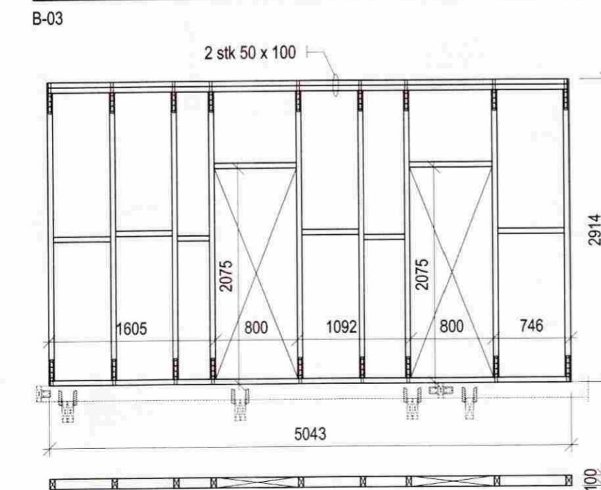
Grind 7 Mkv. 1:50
