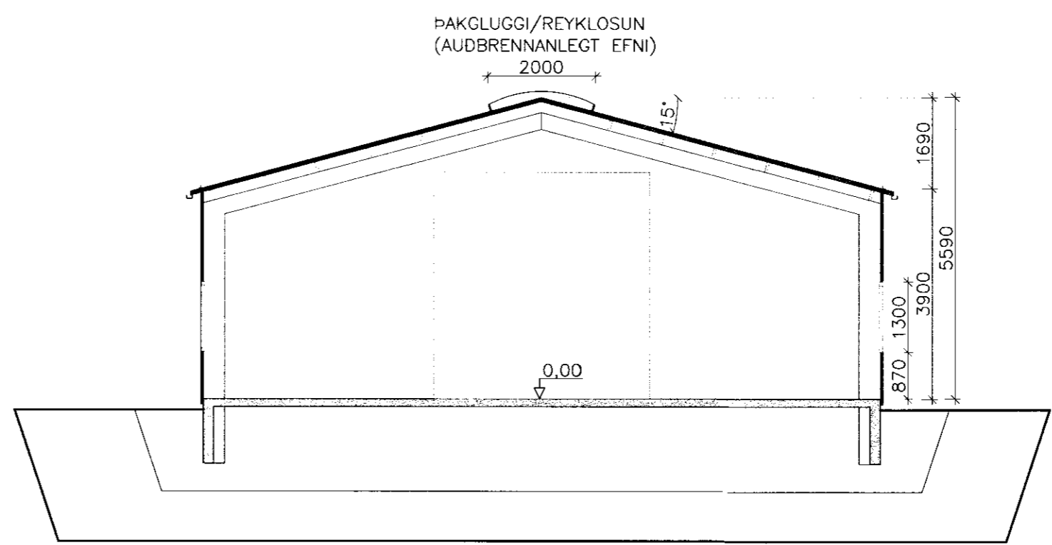
SNEIDING A 1:100
