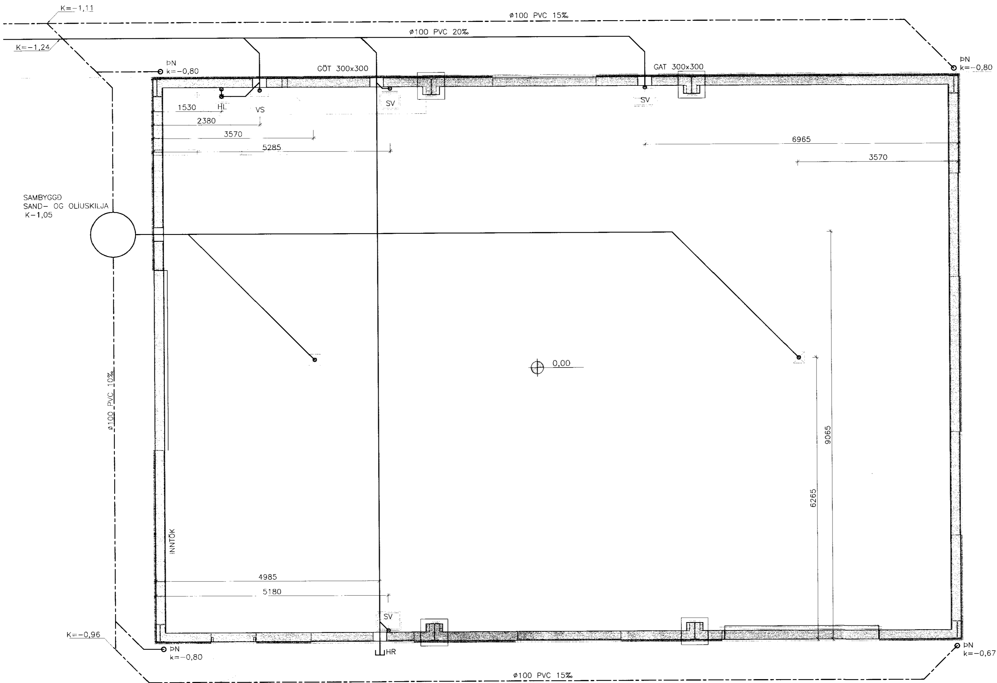
FRÄRENNSLISLAGNIR 1:50
