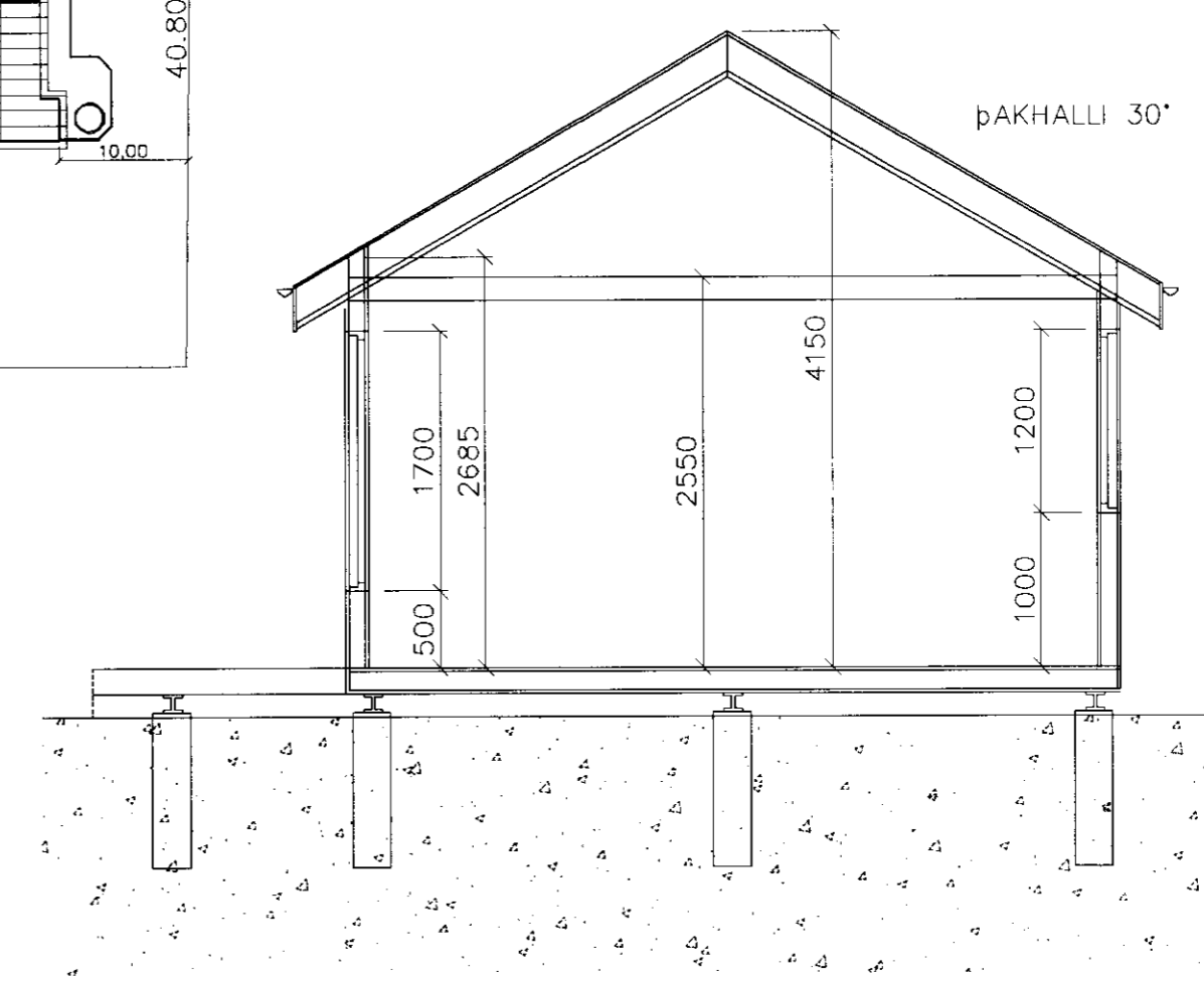
SNÍÐ 1: 50
