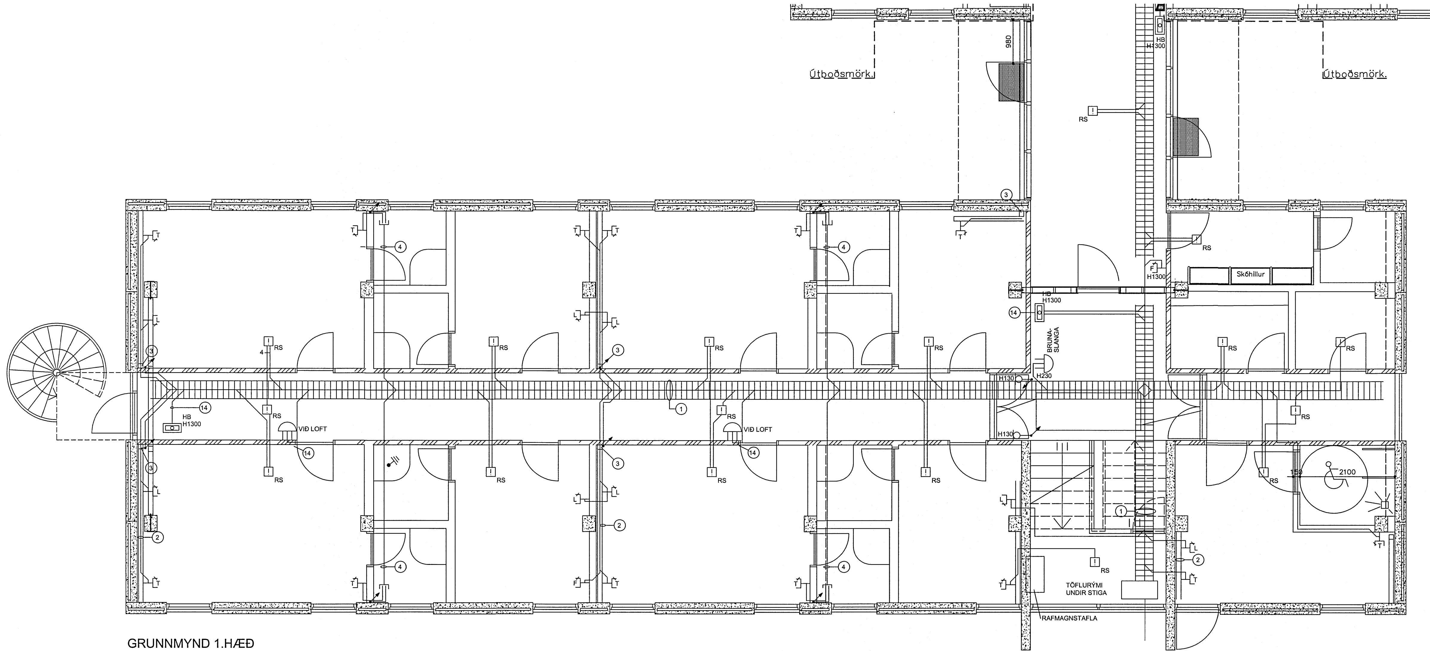
GRUNNMYND 1.HÆÐ
