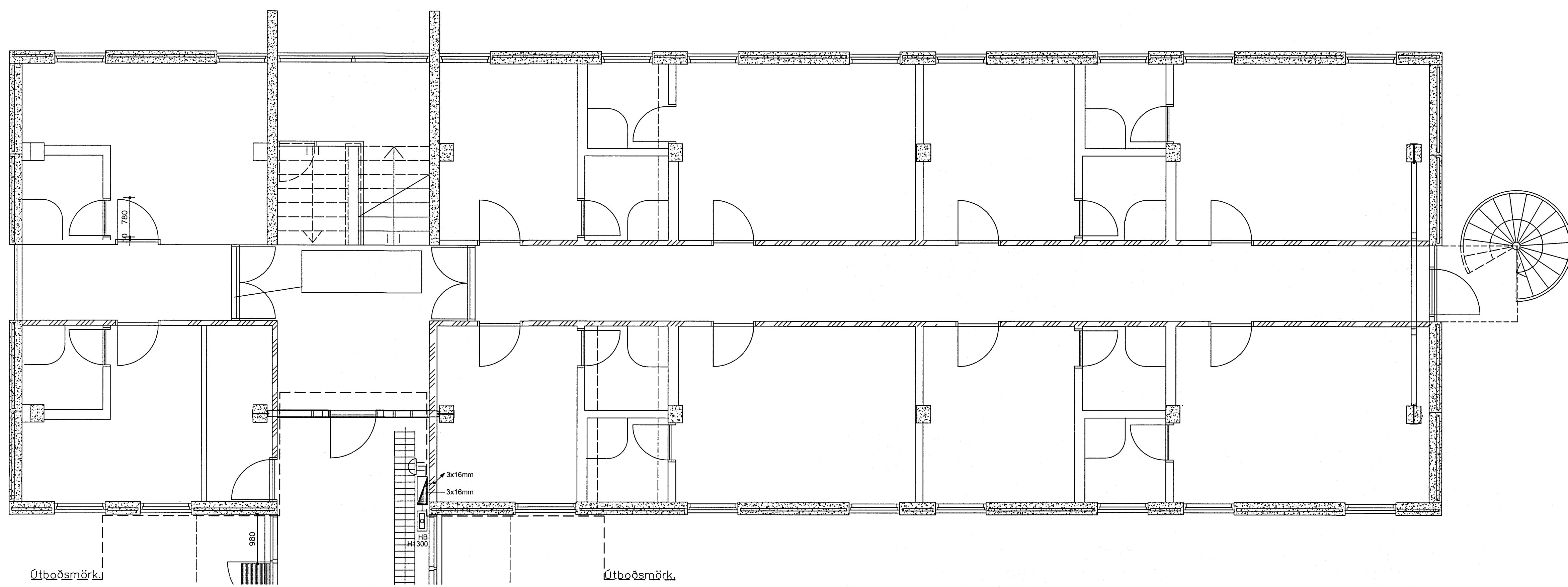
GRUNNMYND 1.HÆÐ
