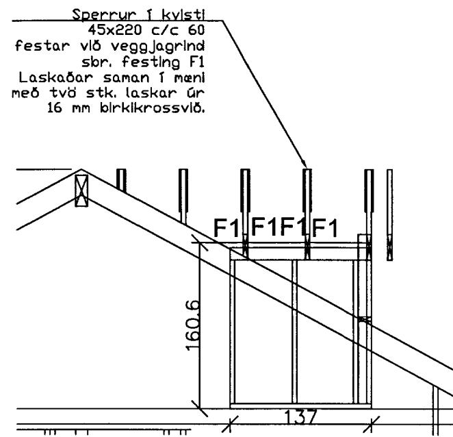
KVISTIR SÉÐ FRÁ HLÍÐ, MKV. 1:20
