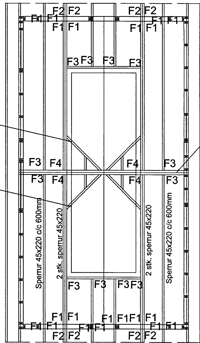
SPERRUPLAN, MKV. 1:50
