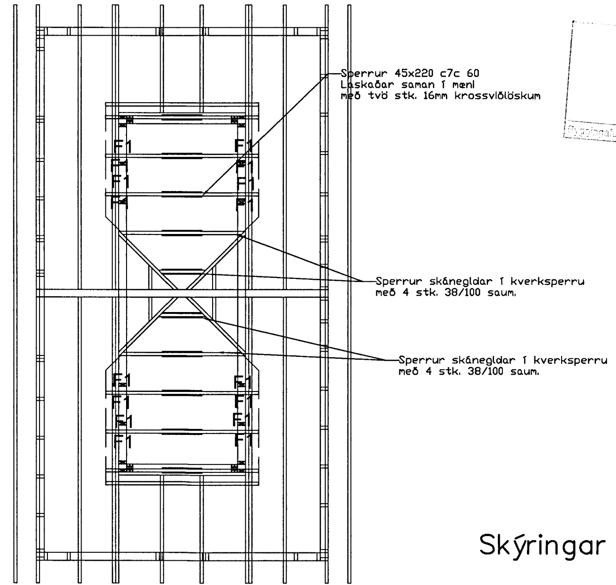
SPERRUPLAN, KVISTIR, MKV. 1:50
