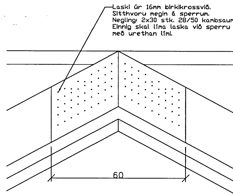
Laskar á mænissamskeytum á kvistsperrum MKV. 1:10
