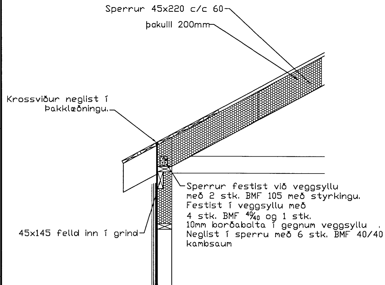
FESTING SPERRA, MKV. 1:20
