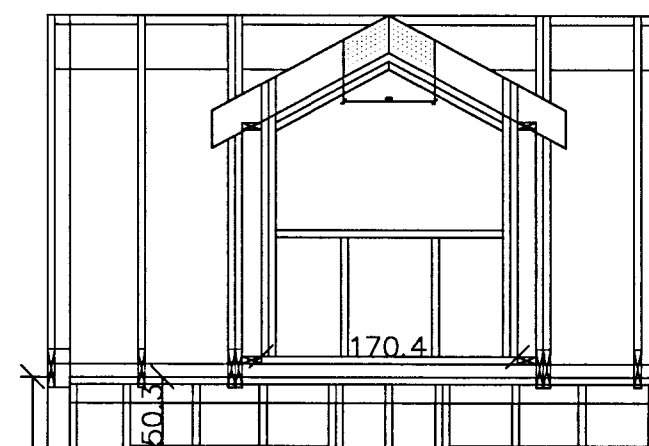
KVISTIR SÉÐAÐ FRAMAN, MKV. 1:20
