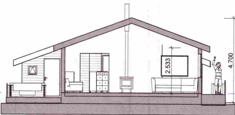
Snið B-B
