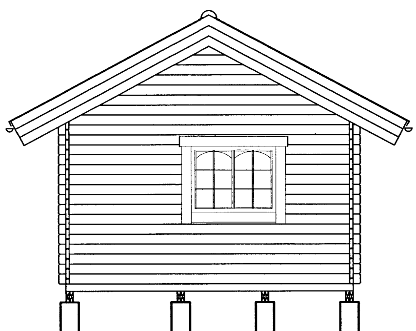
ÚTLIT - AUSTUR
