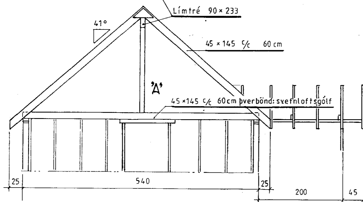
Snið A-A
