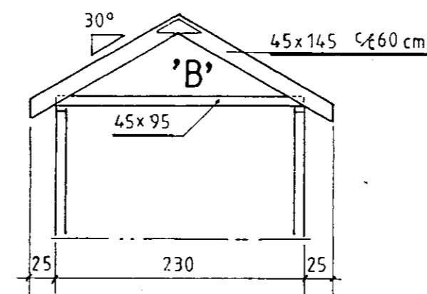
Snið B-B
