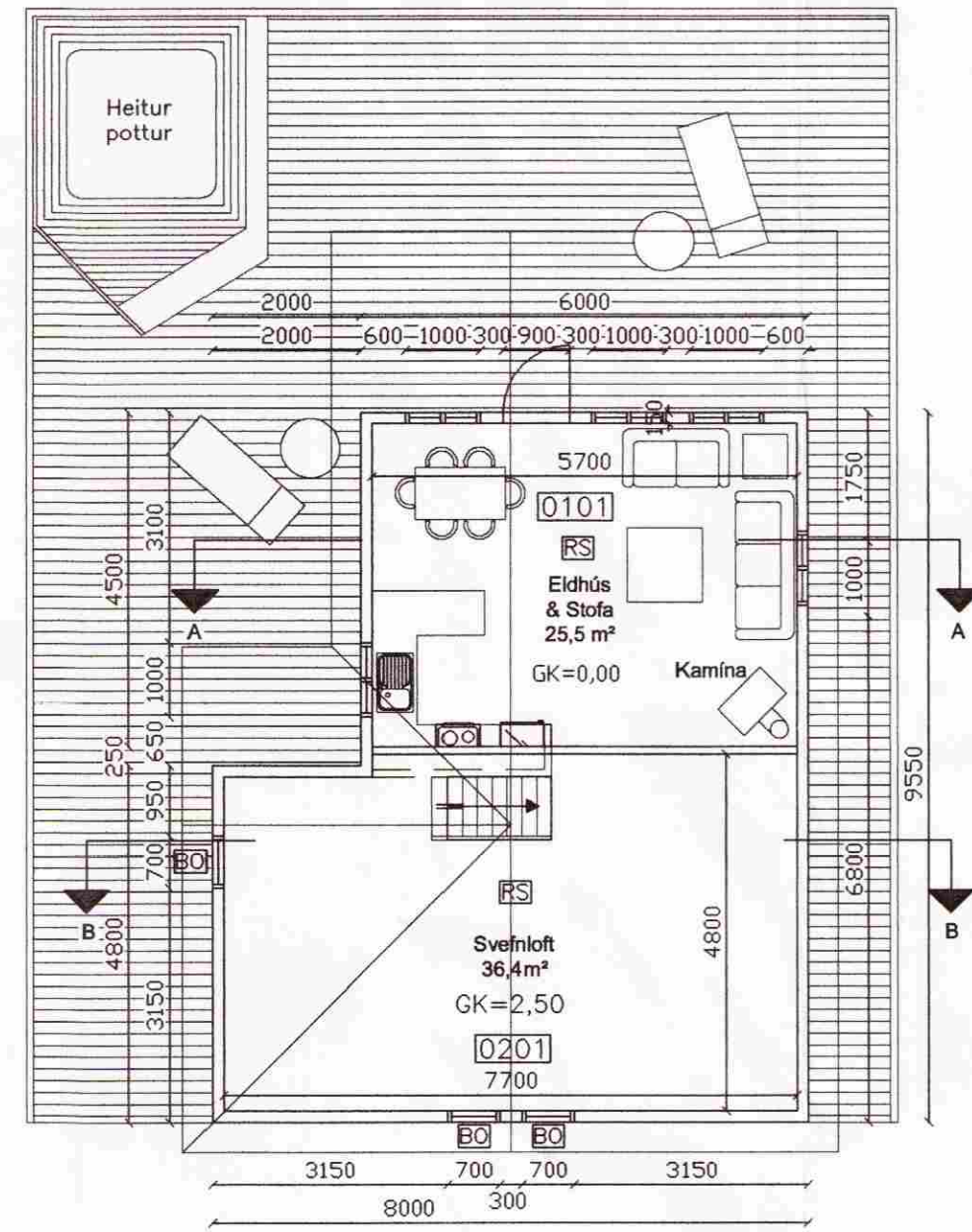
GRUNNMYND, mkv. 1:100
