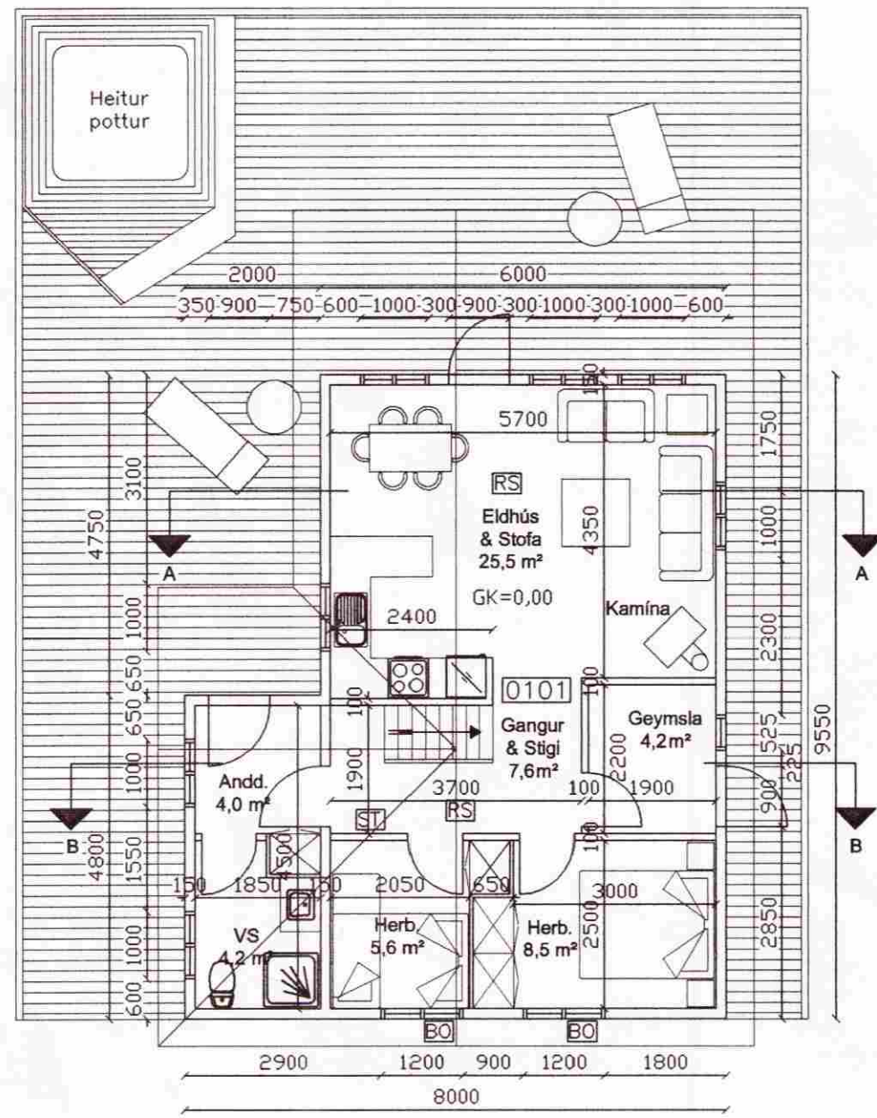
GRUNNMYND, mkv. 1:100
