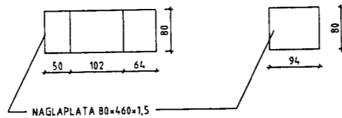
NAGLAPLATA 80x460x1,5
