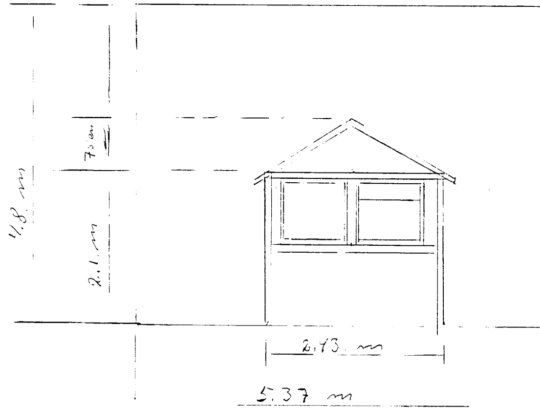
NORÐUR HLIÐ
