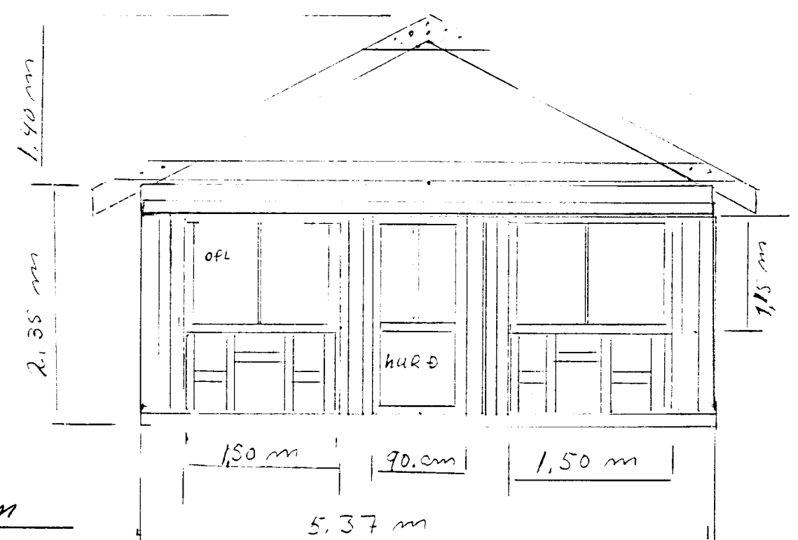
SÚÐUR HLIÐ
