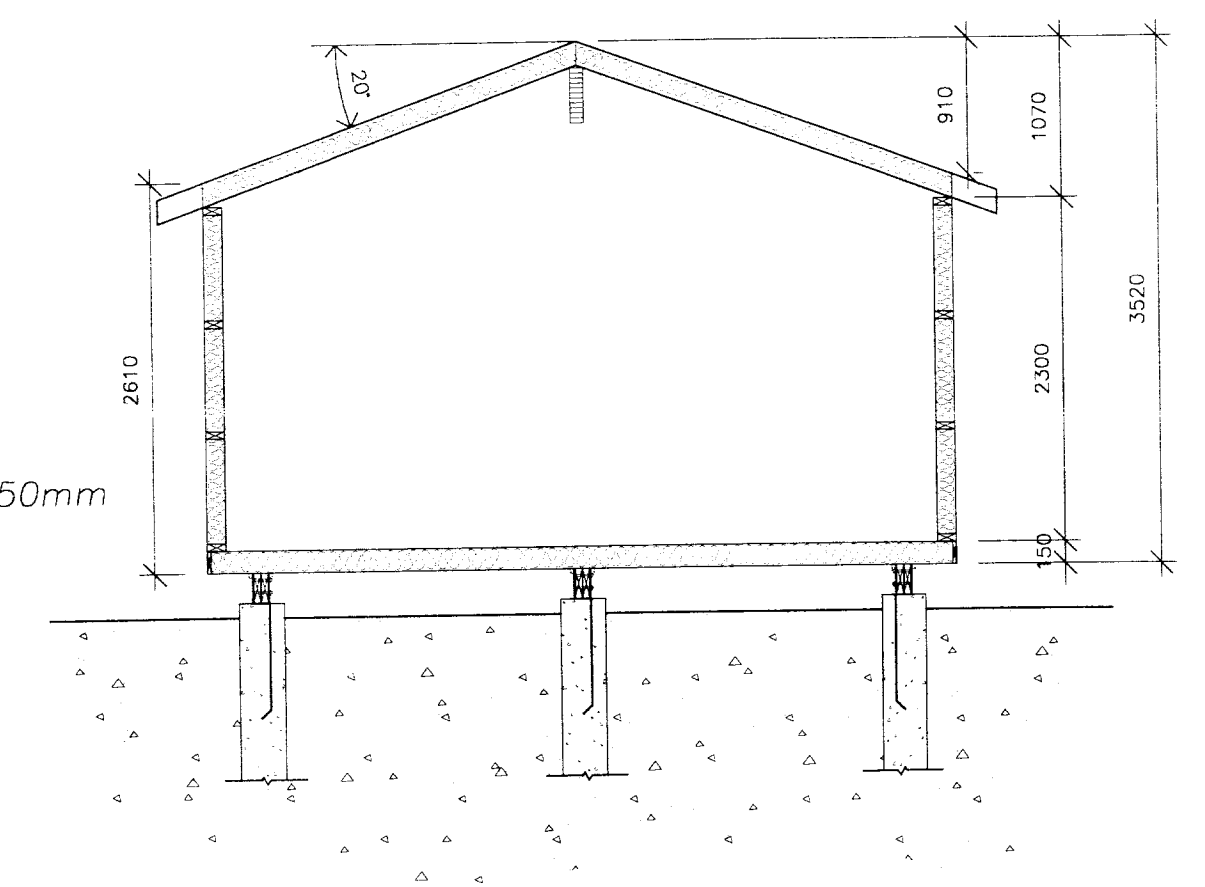
Snið AA Málkvarði 1:50
