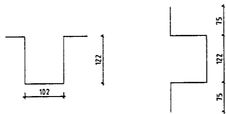
F1 M 1:5
