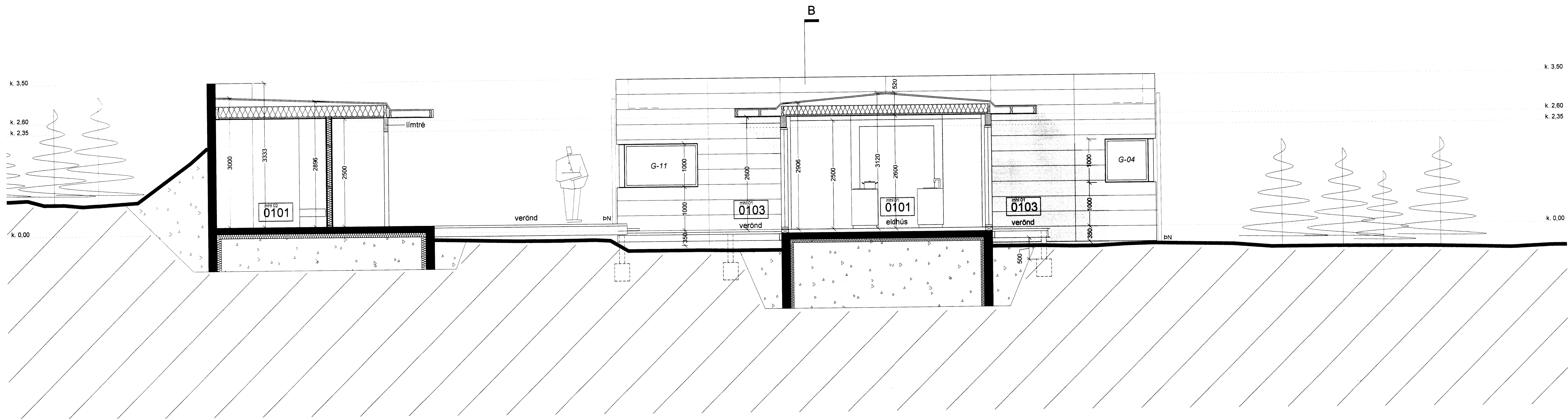
SNEIÐING A - A M 1:50
