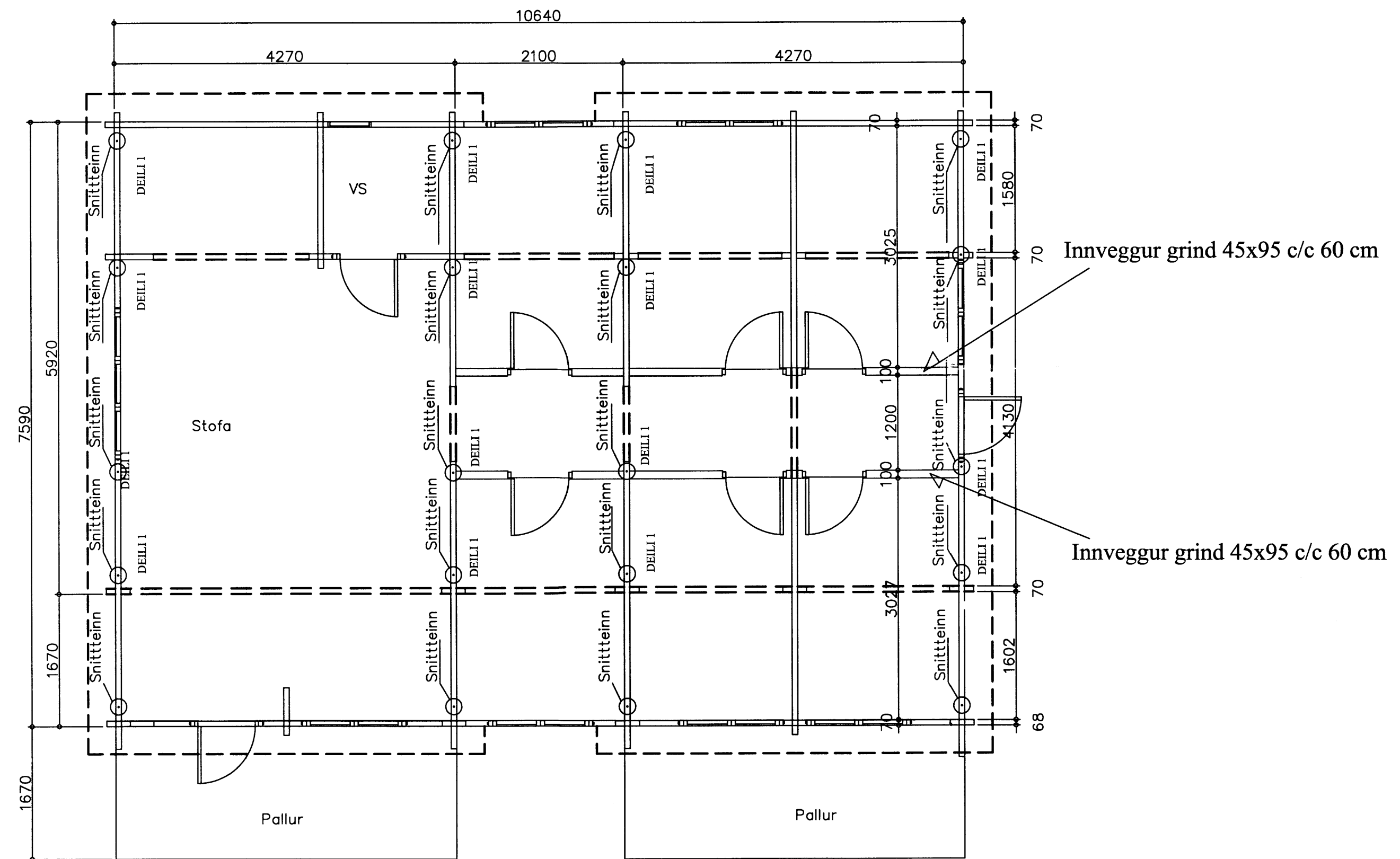
Grunnmynd út og innveggir
