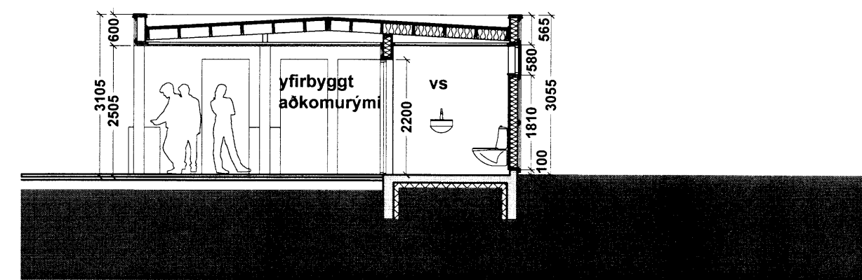
Snið A-A mkv 1:100
