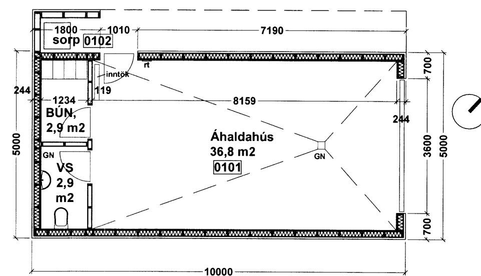
Grunnmynd mkv 1:100
