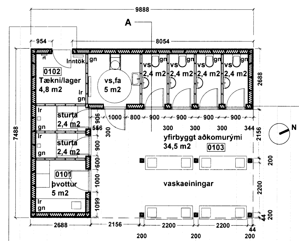
Grunnmynd mkv 1:100
