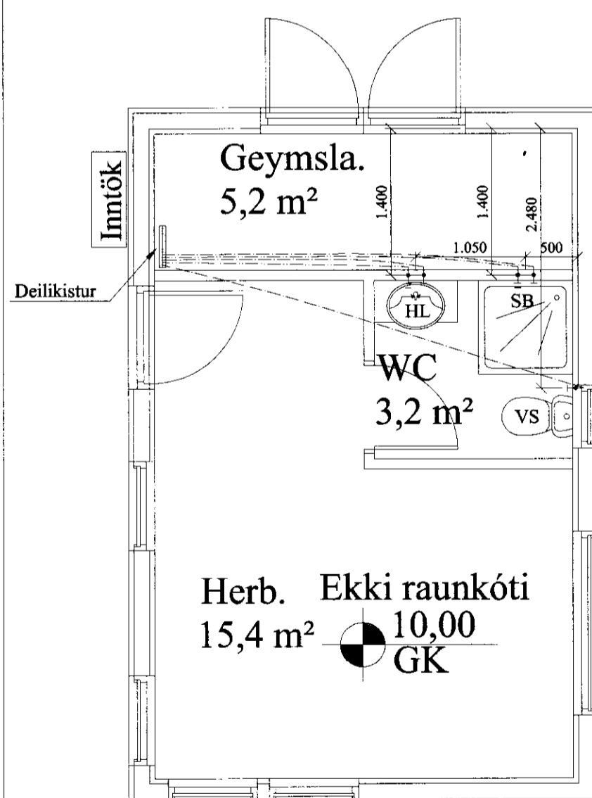
Grunnmynd neysluvatnslagna mkv. 1:50
