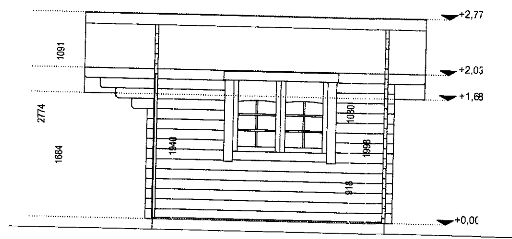
Snið A-A 1:50
