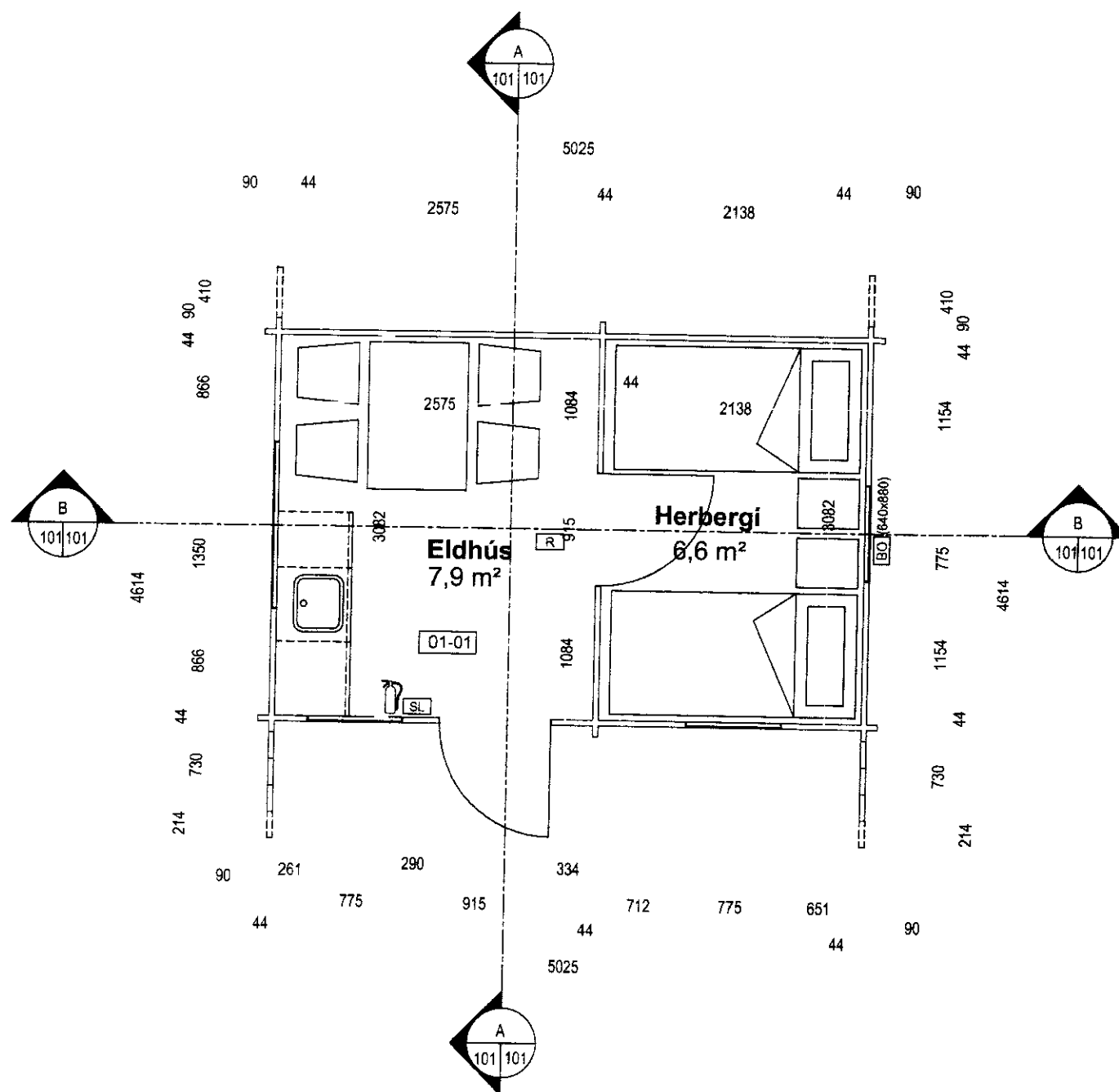
Grunnmynd 1:50
