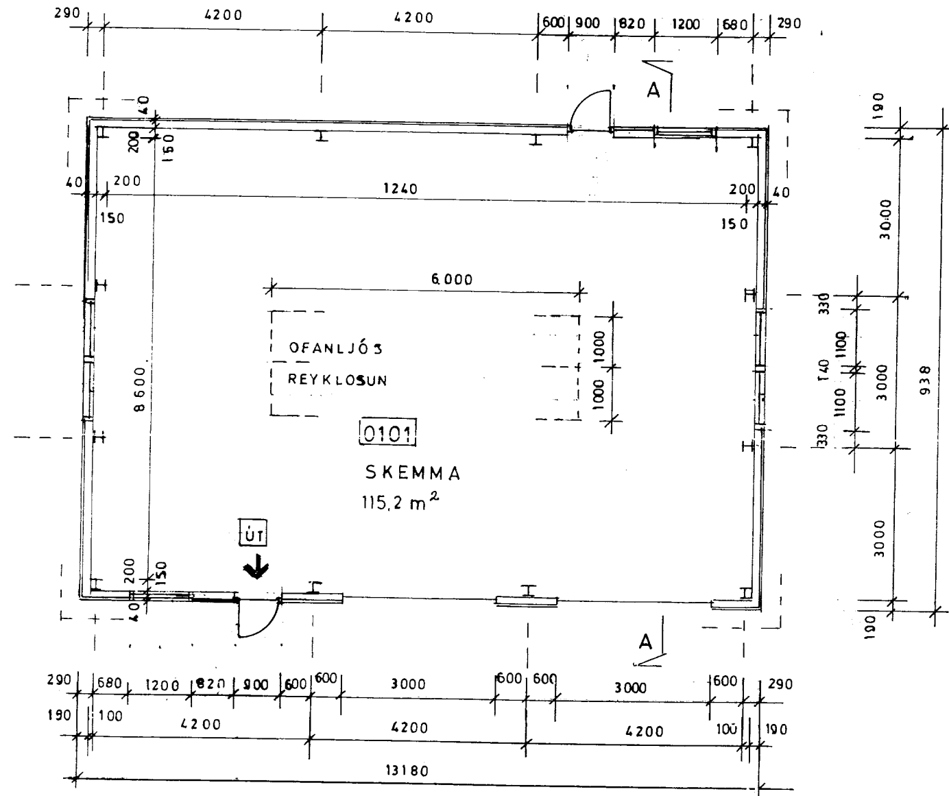
grunnmynd
