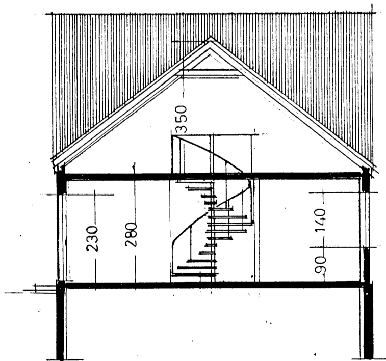
SKURÐUR
