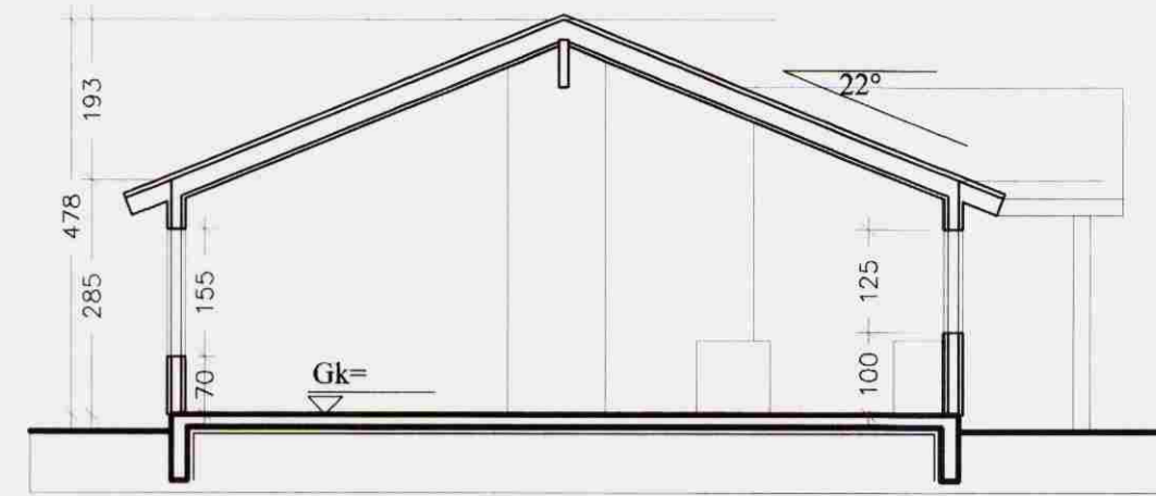
SNEIÐING a-a 1:100
