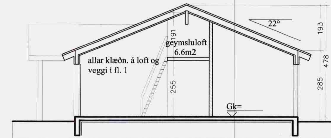
SNEIÐING b-b 1:100
