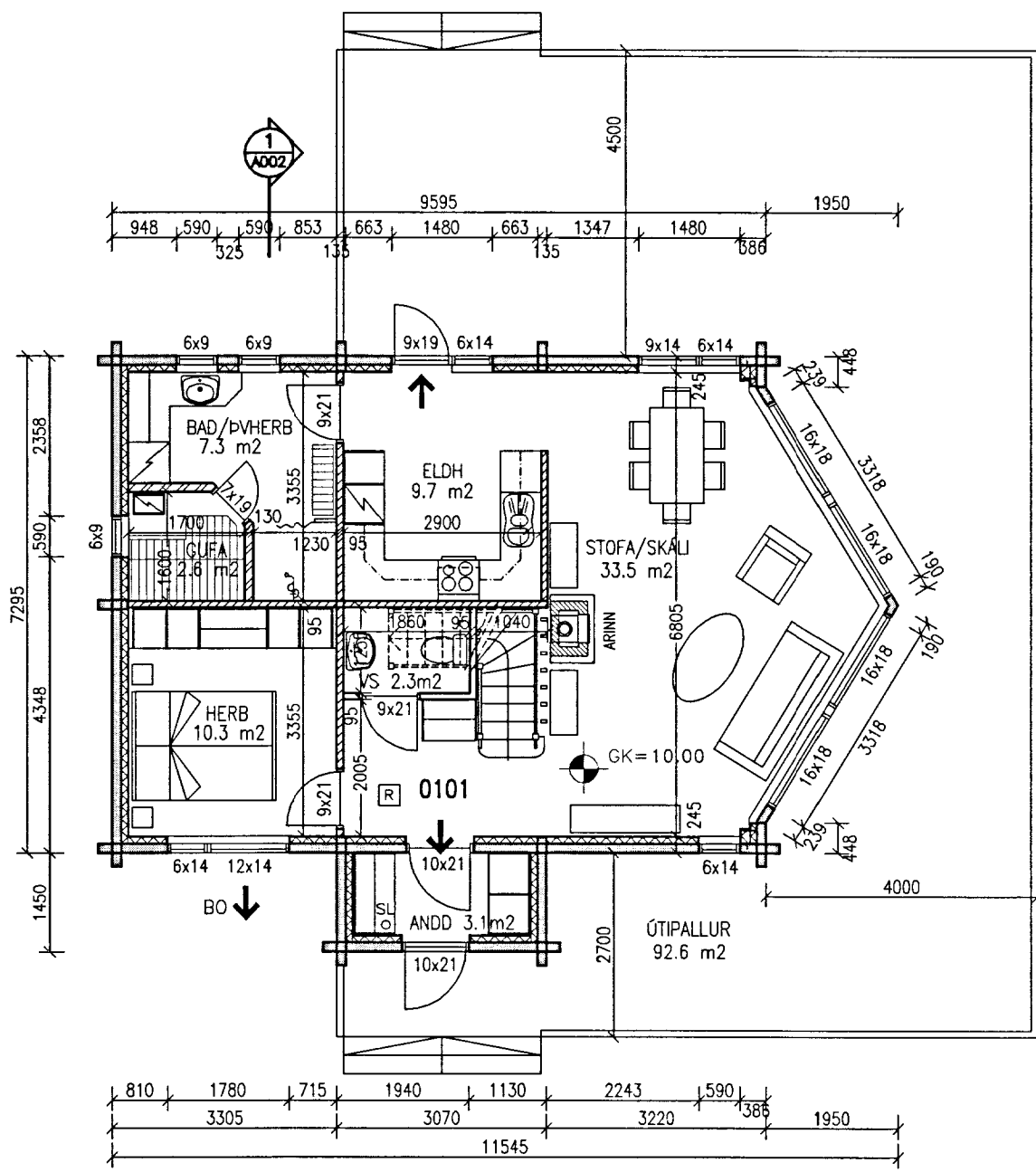
GRUNNMYND 1. hæð 1:100
