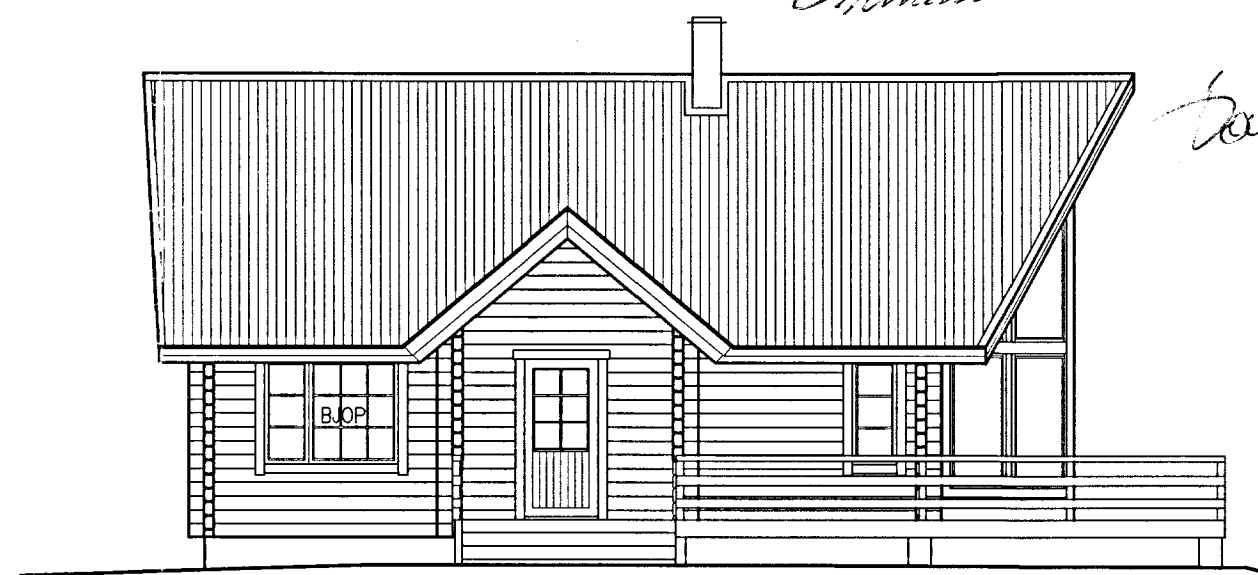
ÚTLIT NORDVESTURHLIÐ
