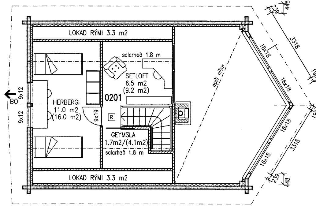
GRUNNMYND 2. hæð 1:100
