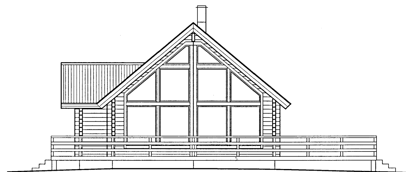
ÚTLIT SUDVESTURHLIÐ
