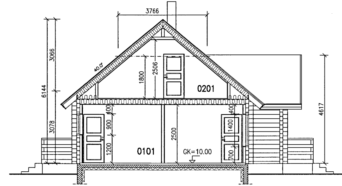
SNID 1-1 1:100
