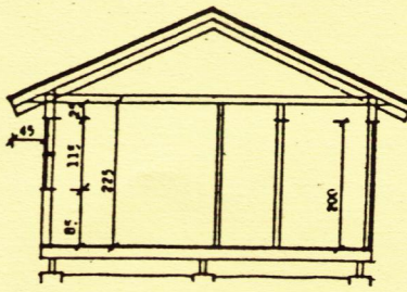
500 SNEIÐING
