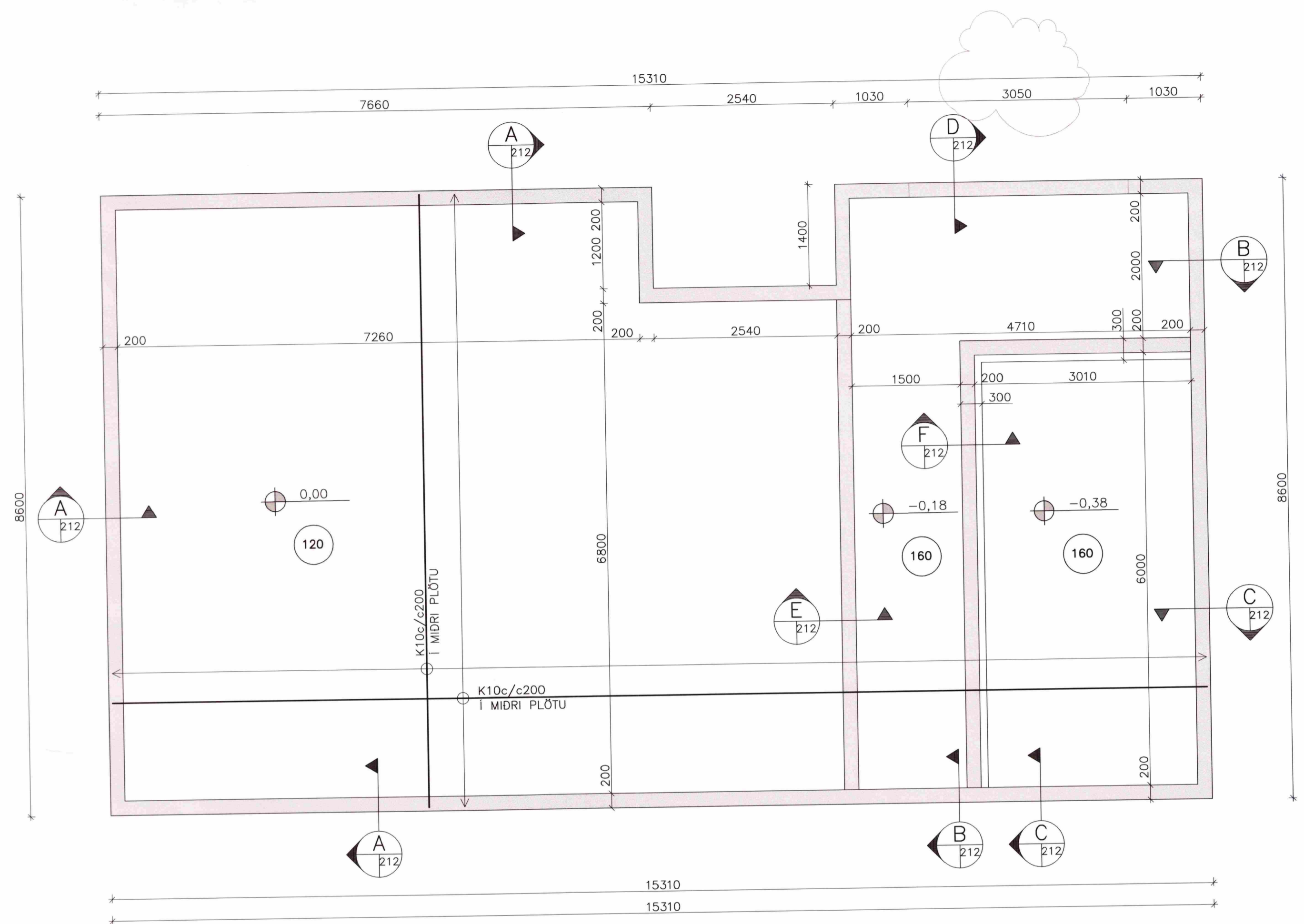
UNDIRSTÖÐUR GRUNNMYND 1:50
