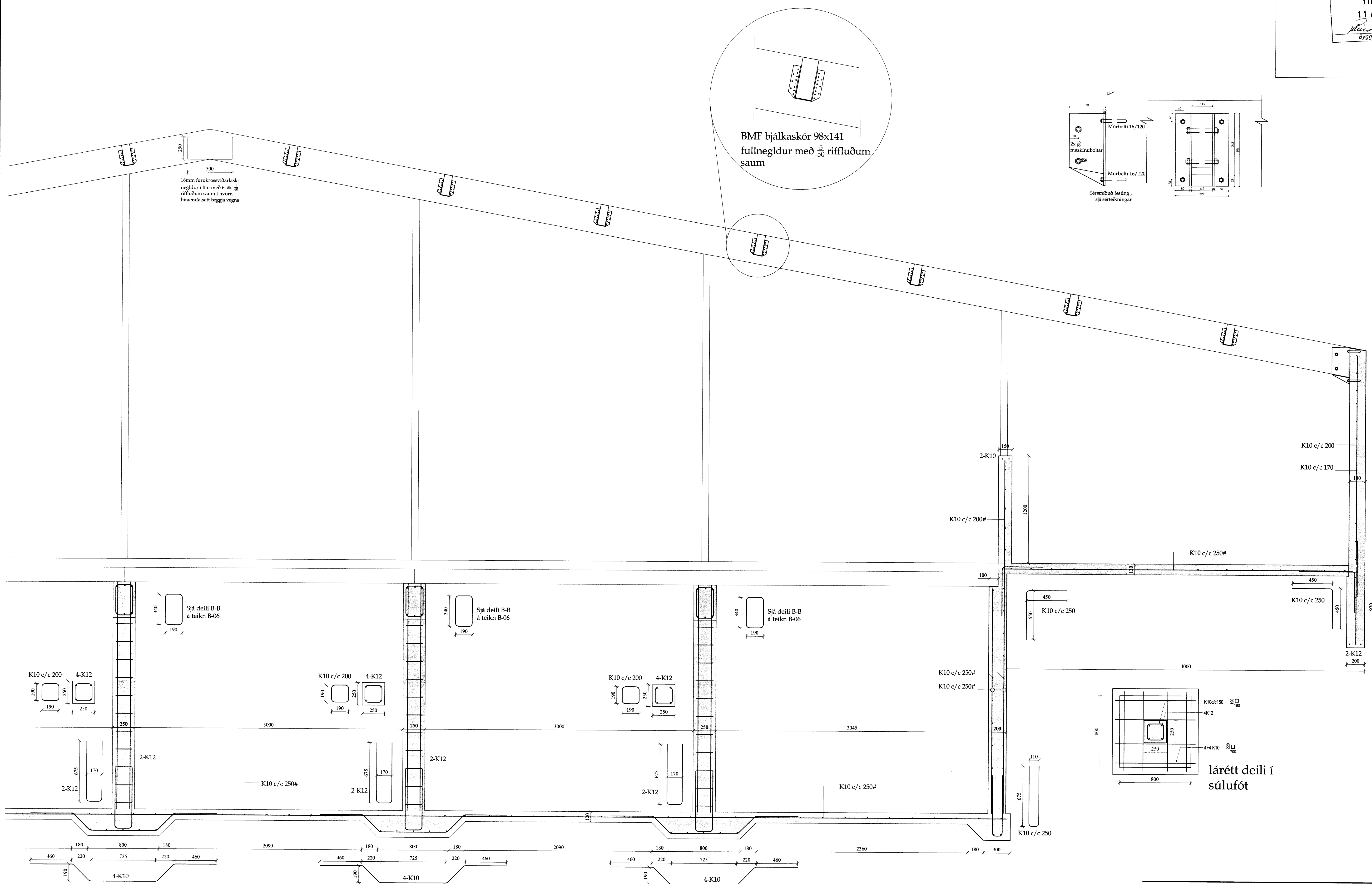
Pverdeili A-A mk. 1:20 (teikn B-01).Seinni hluti
