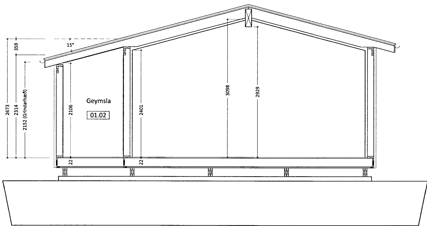
SNID B-B Mkv. 1:50
