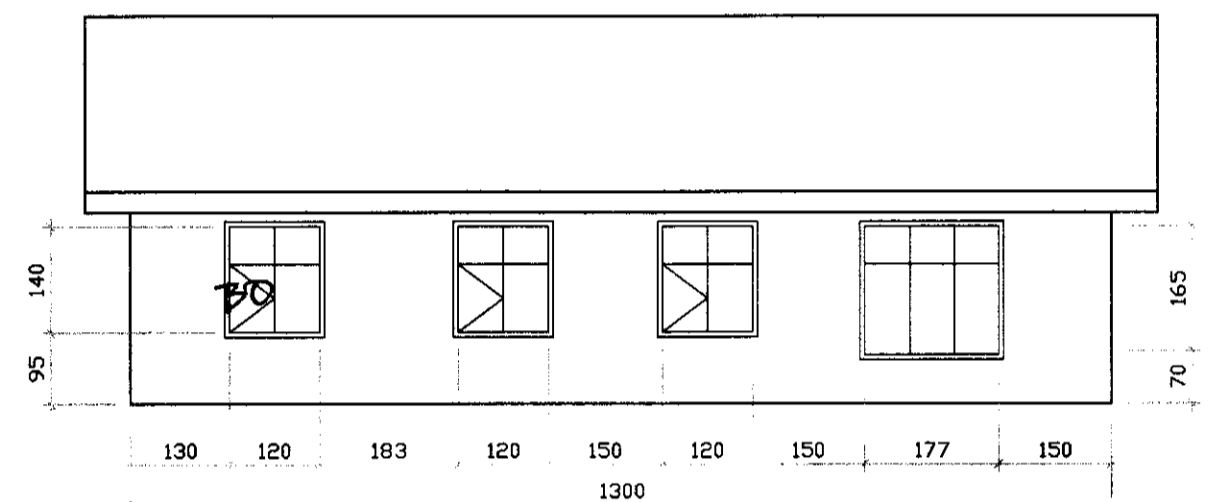
Útlit - austur 1:100
