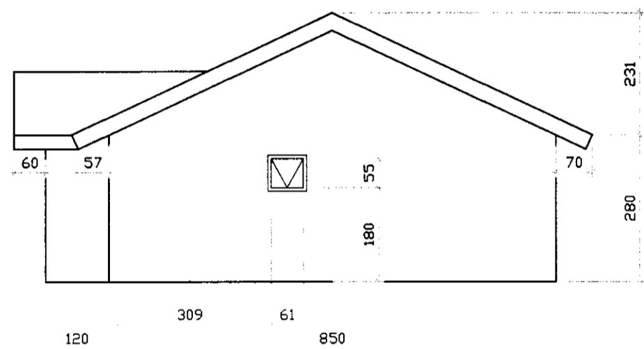
Útlit - suður 1:100
