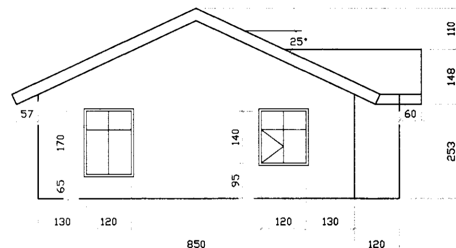
Útlit - norður 1:100
