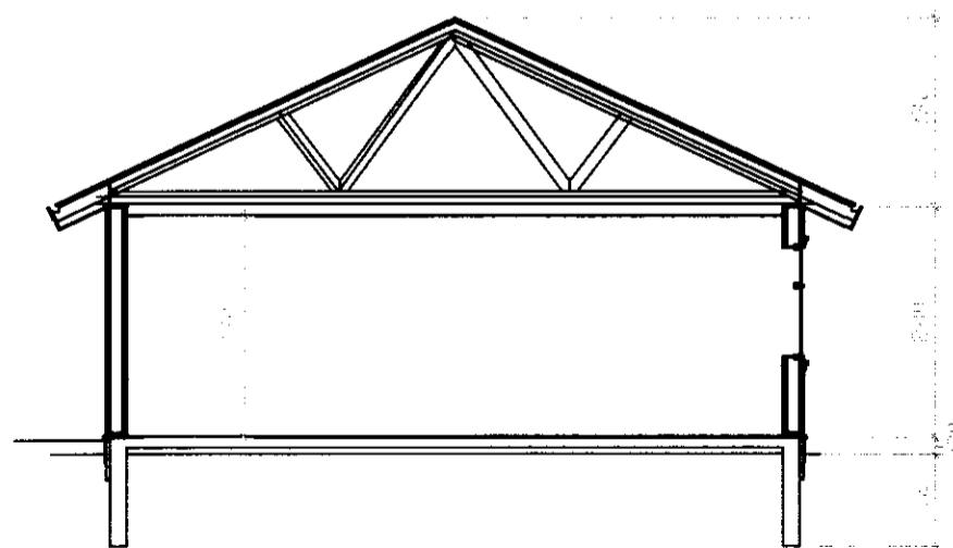
Snið A-A 1:100
