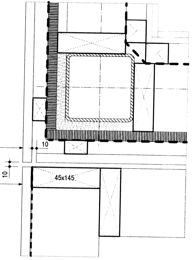
8 DEILI - HORN VIÐ HÚS 1:20
