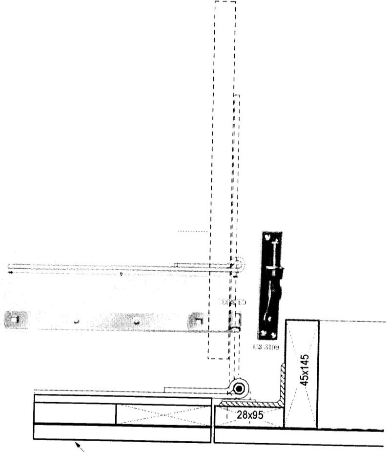
3 DEILI - ÞAK VIÐ HÚS 1:20
