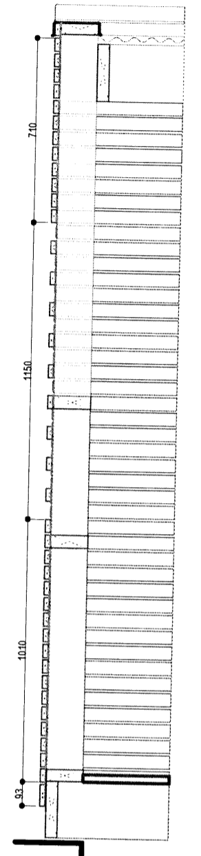
1 SNEIÐING - UPPBYGGING 1:20
