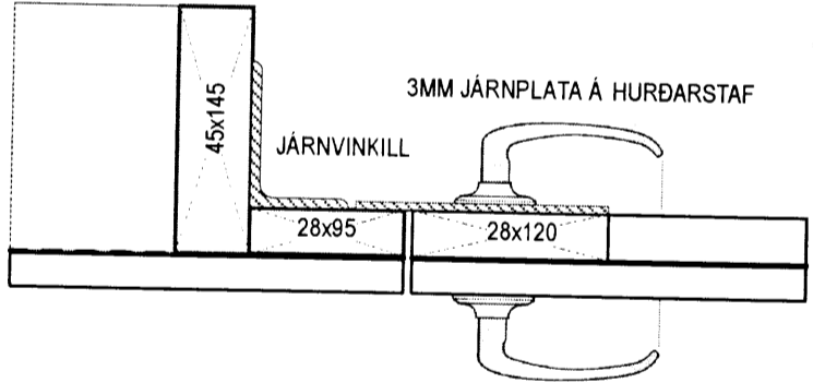
6 DEILI - HJALLUR HURÐ / HLERI 1:20
