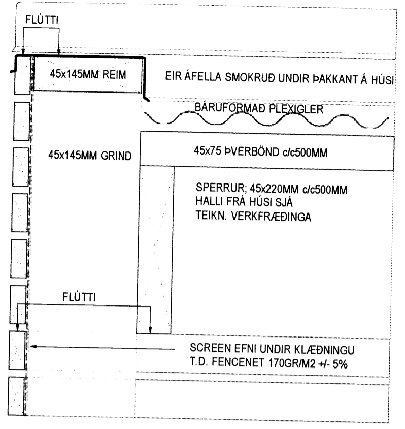
4 DEILI - ÞAKFRÁGANGUR, HLIÐAR 1:20
