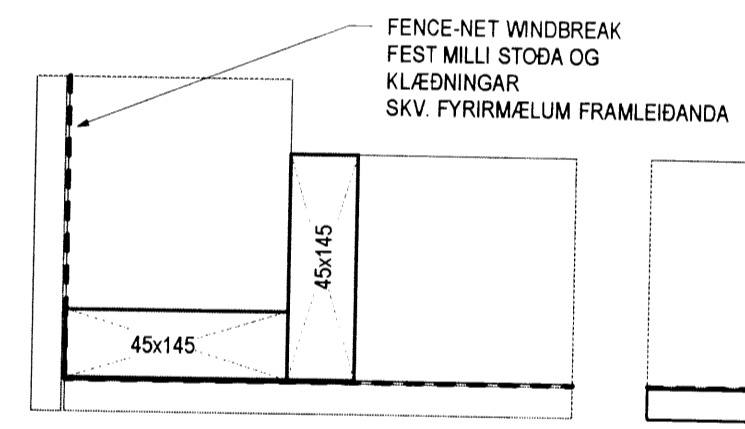
8 DEILI - HORN VIÐ HÚS 1:20
