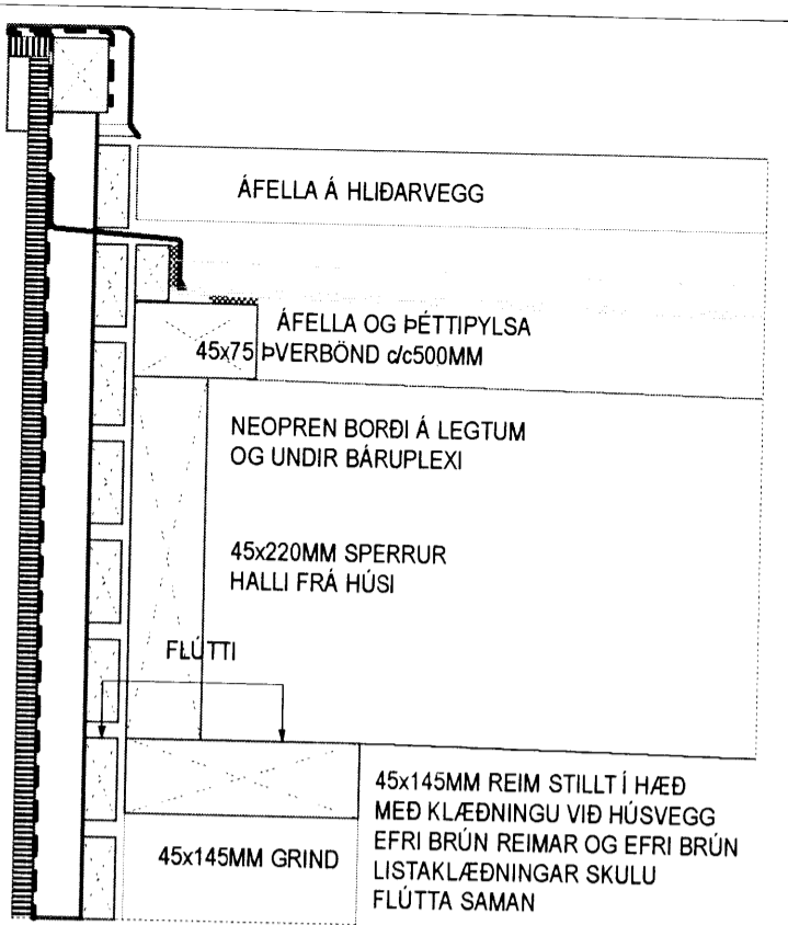
3 DEILI - ÞAK VIÐ HÚS 1:20
