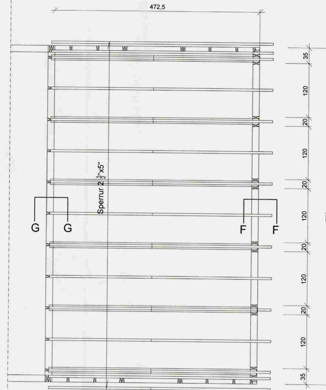
Grunnmynd 1:50, þakviðir - syðri endi
