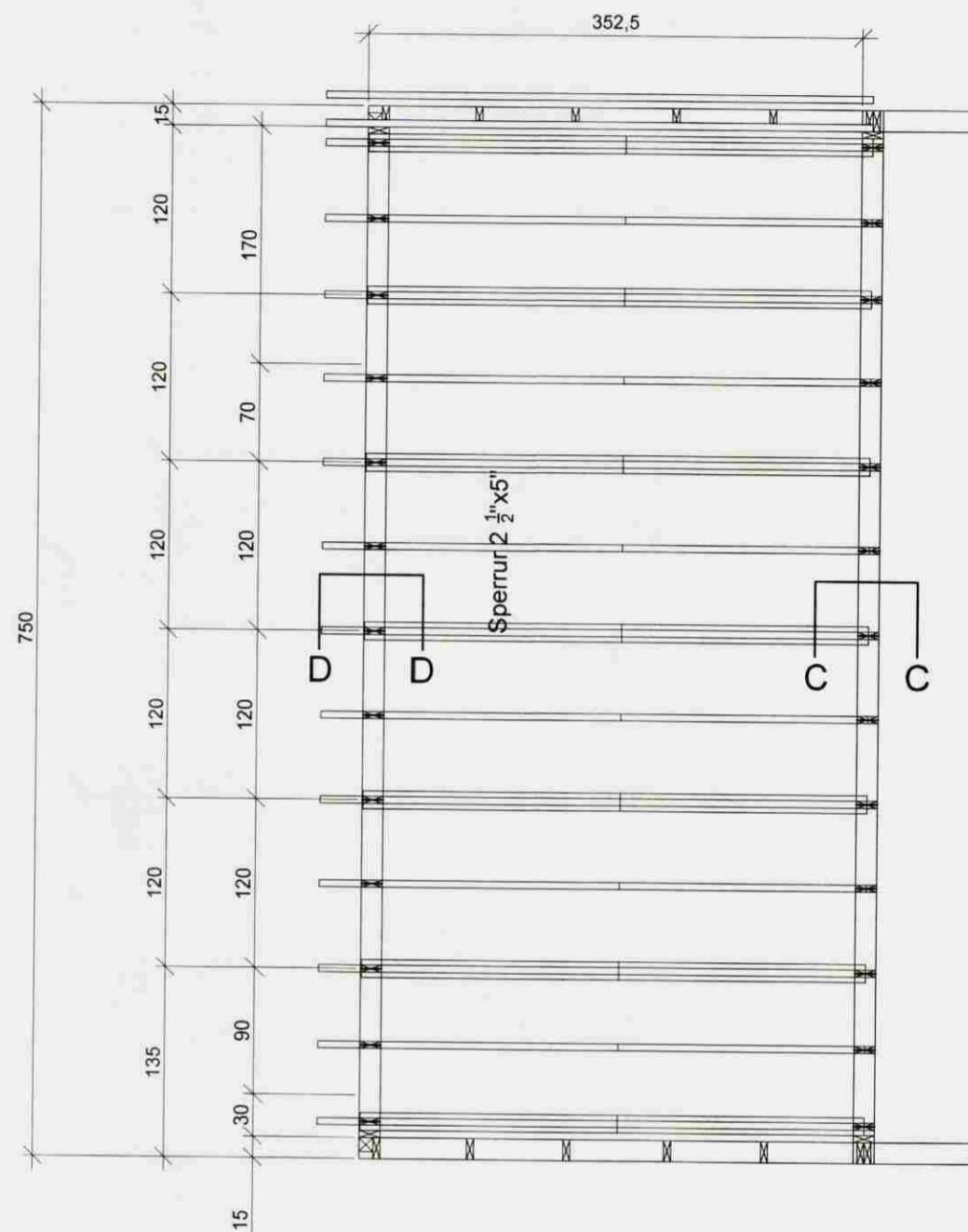
Grunnmynd 1:50, þakviðir - norður endi
