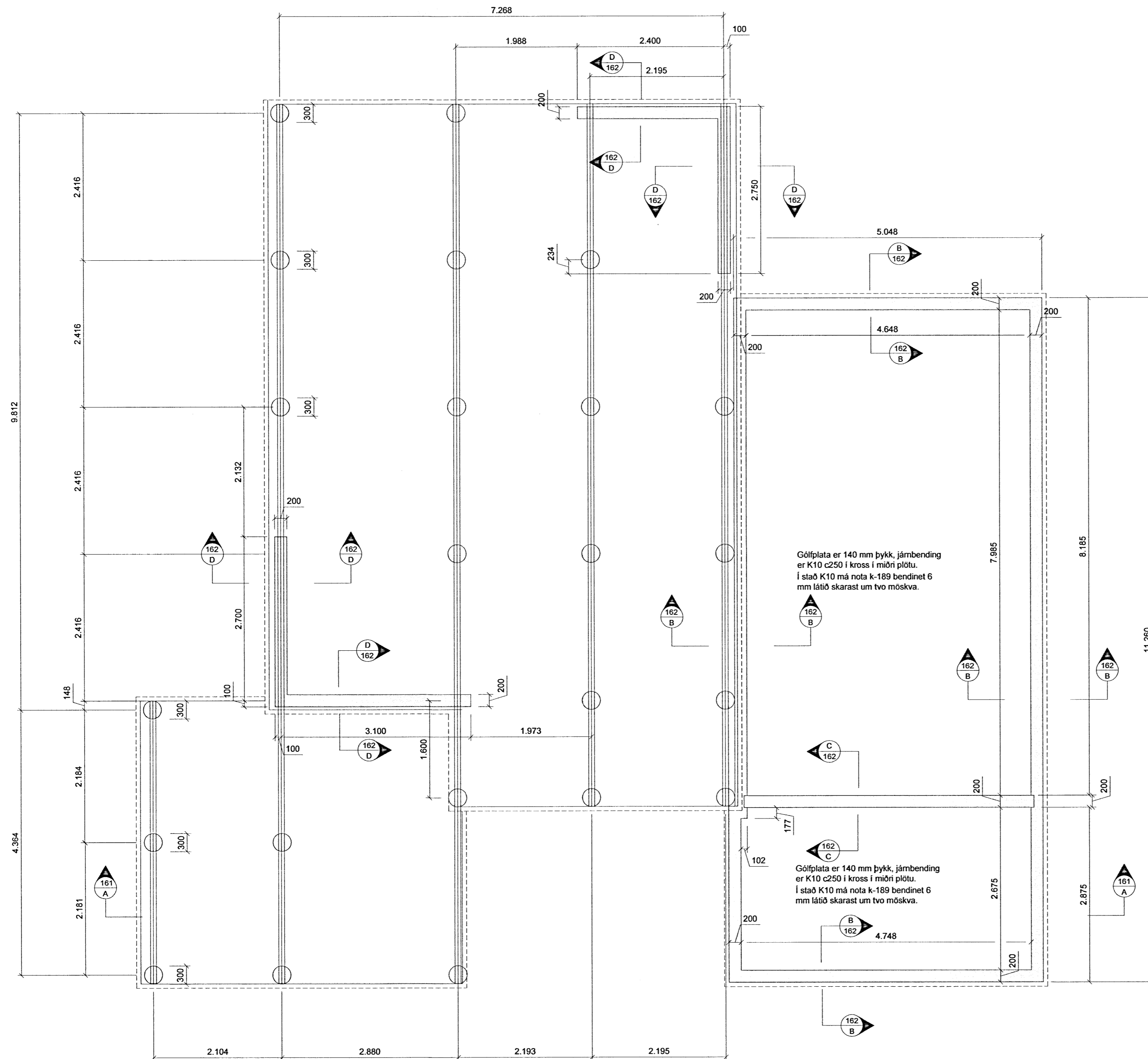
Grunnmynd sökkla og súluplan mkv. 1:50
