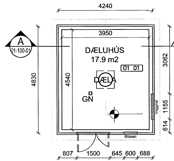
Grunnmynd
