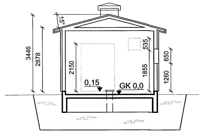
Snið A
