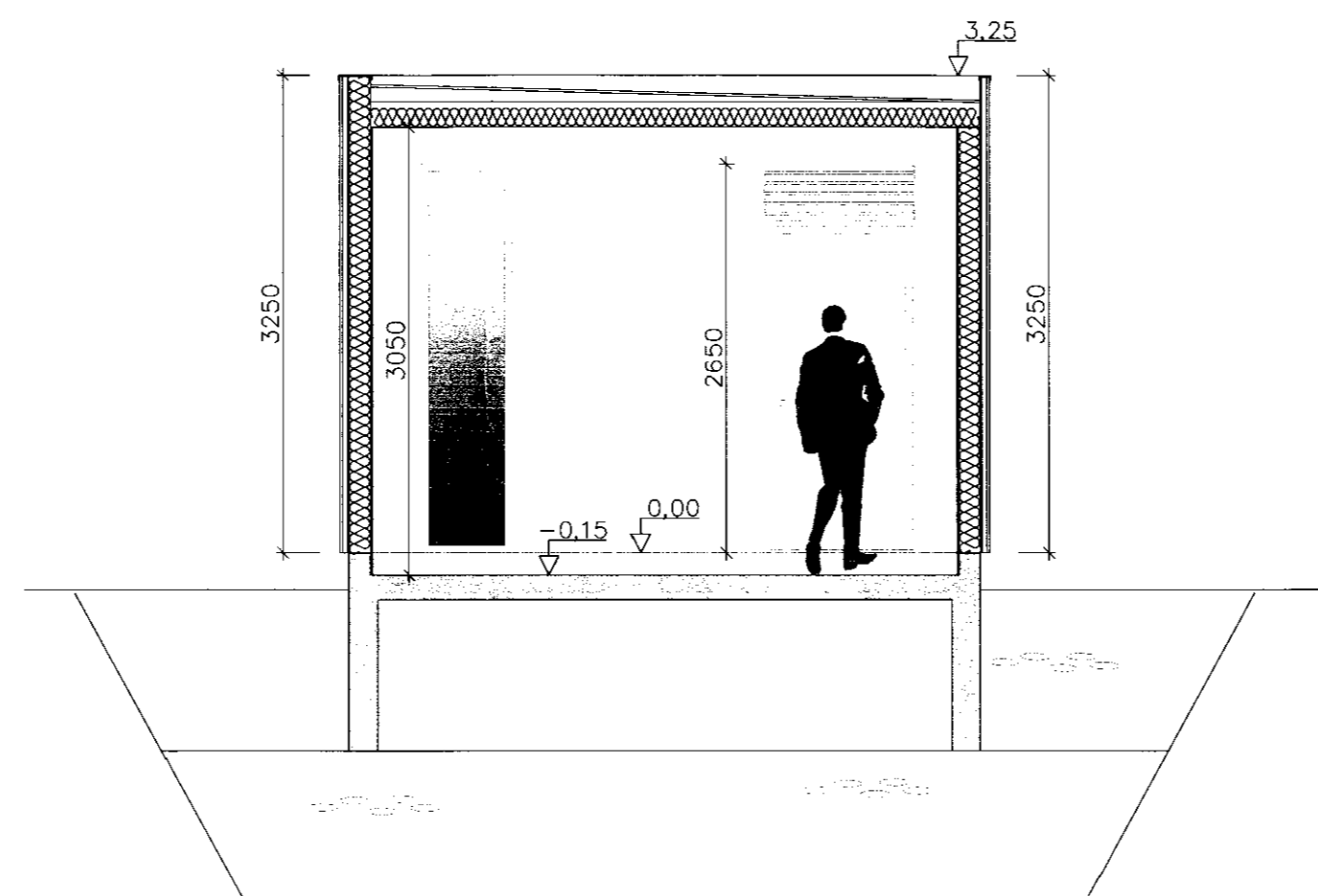
SNEIDING A-A 1:50
