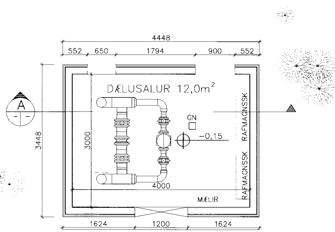
GRUNNMYND 1:50
