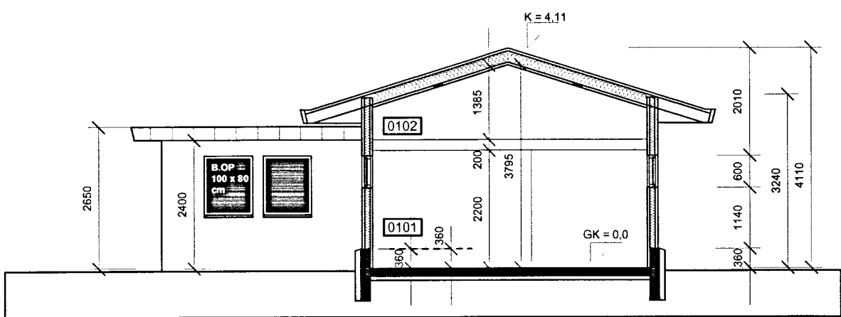
SNEIÐING M 1:100
