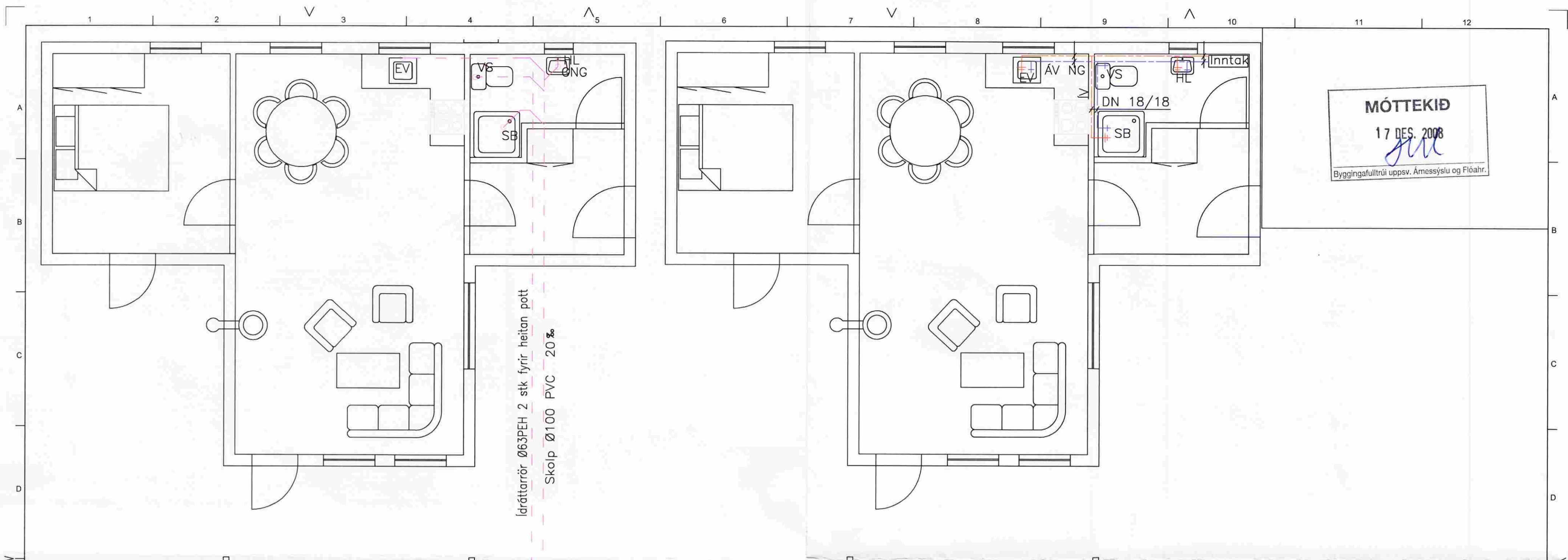
Grunnmynd fráveitulagna 1:50
