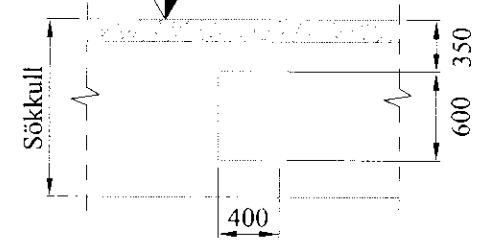
Skýringamynd af inntaksgati GK: 00,00
