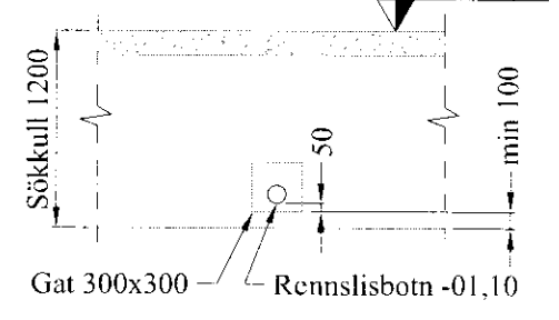
Skýringamynd af inntaksgati GK: 00,00
