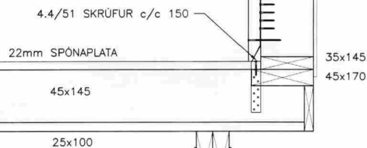
FESTING LANGHLIDAREININGA VID GÓLFBITA: MKV. 1:10 BMF 48x320 GAFFALJARN NEGLIST MED 2x8 STK. KS 31/40 Í STODIR OG GÓLFBITA
