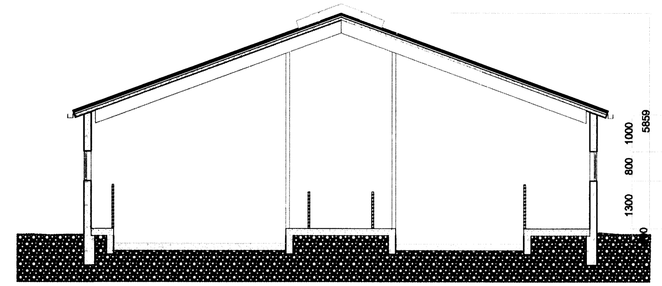
Snið S - 01
