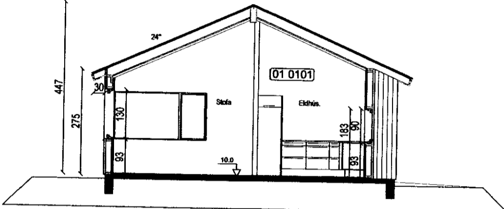
Snið B-B Mkv 1:100
